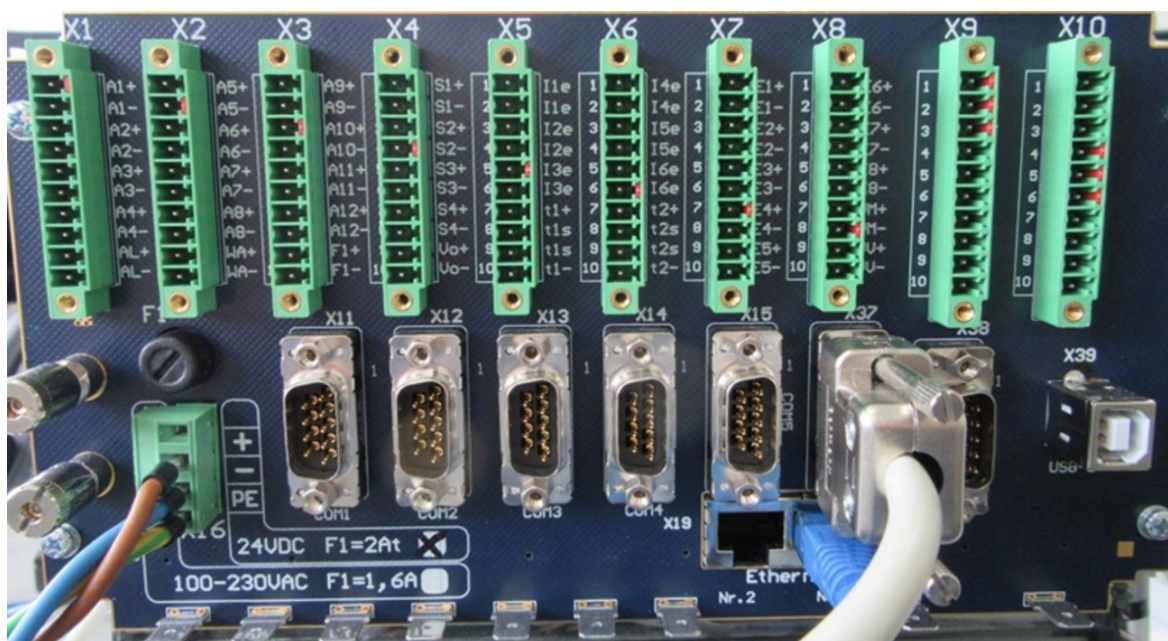
Fig. 8.20: Collegamento dell'interfaccia Modbus dell'USM a COM 6
