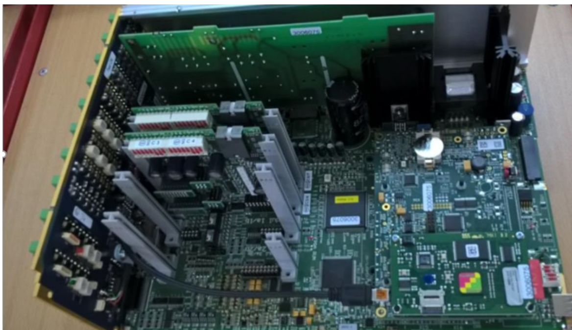
Fig. 8.7: Slot per COM6 e 7 dell'ERZ 2000-NG
