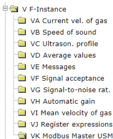
Fig. 8.18: Sottodirectory menu V di Instanz-F in ERZ2000-NG
