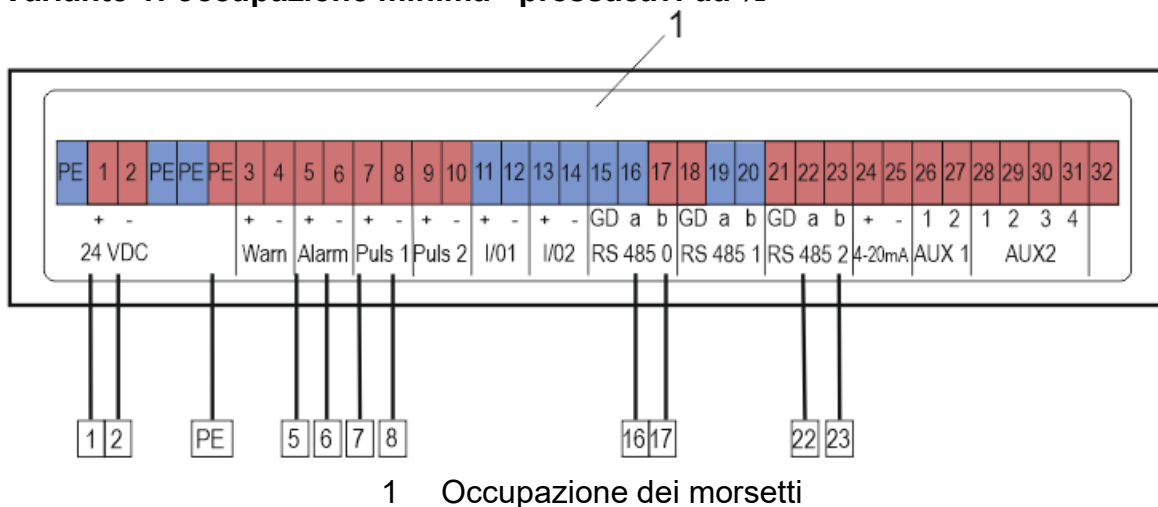
Fig. 8.9: Collegamento con pressacavi da ½" e 11 fili misura AWG 18 (consentiti max. 11; Killark tipo ENY-1TM).
