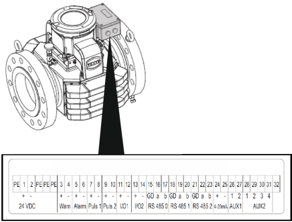
Fig. 8.7: Occupazione dei collegamenti sulla morsettiera
