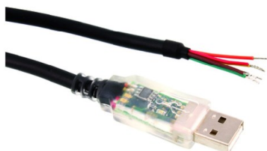
Fig. 8.40: TIPO USB-RS485-WE-1800-BT 687-7834 (1,8 m) o Tipo USB-RS485-WE-5000-BT 730-0164 (5,0 m)
