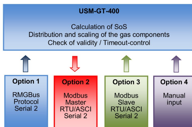
Fig. 4.3: Importazione dei dati di analisi dei gas
