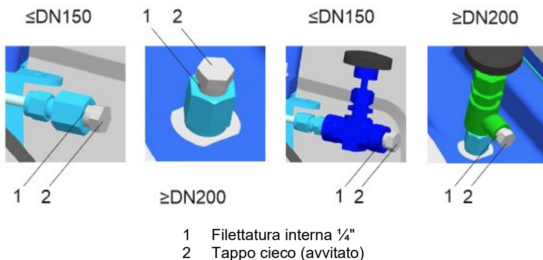
Fig. 8.25: Possibilità di connessione del collegamento in pressione con filettatura interna
