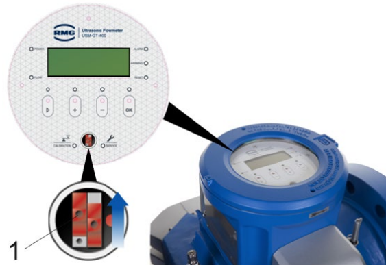
1 Eichschalter
