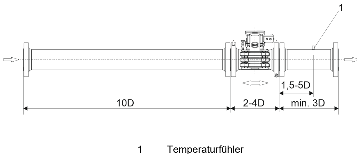
Abb. 7.4: Unidirektionaler Betrieb
