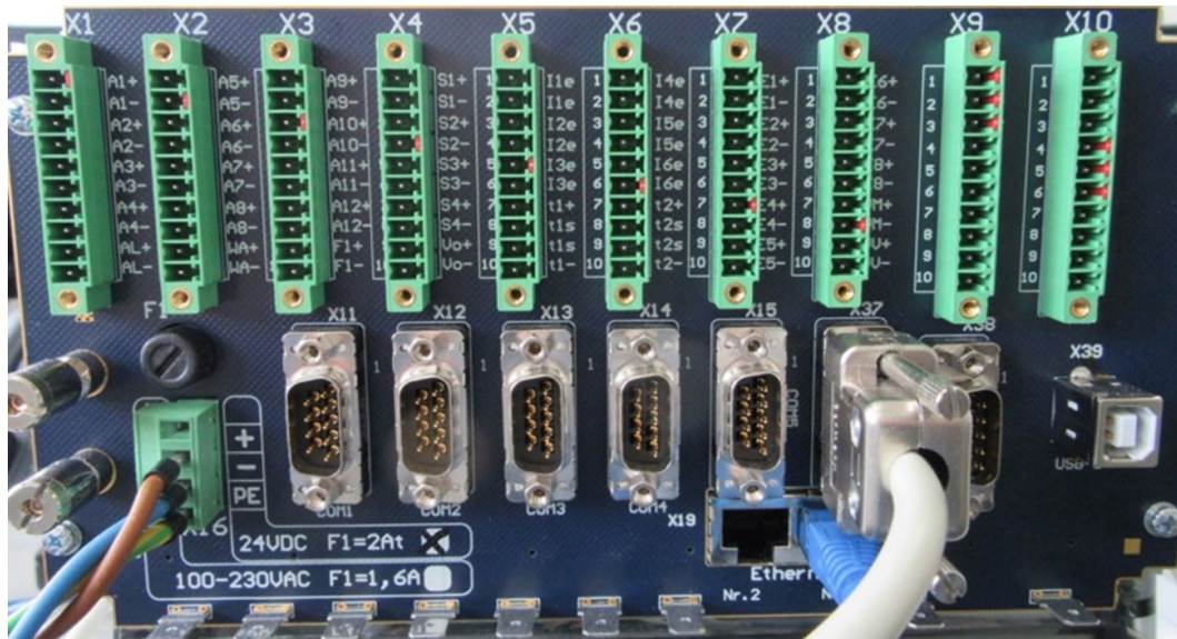
Abb. 8.18: Anschluss der Modbus-Schnittstelle des USM an COM 6
