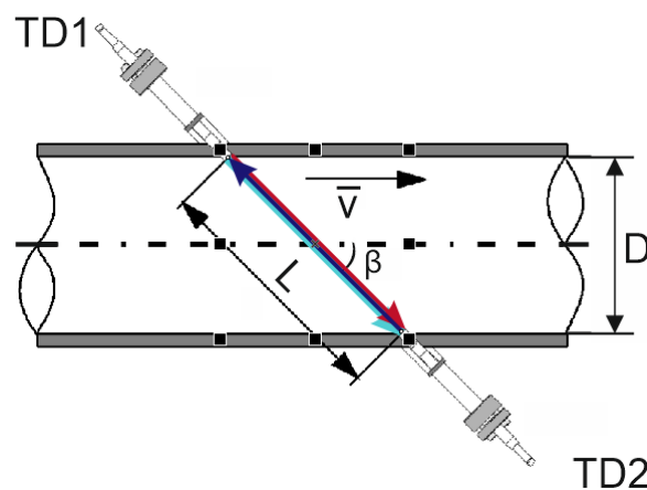
Abb. 4.2: Erweiterte Schallgeschwindigkeitsmessung
