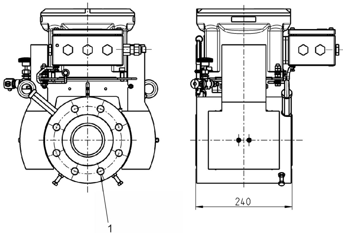
Abb. 13.7: Gewichte und Maße DN80
