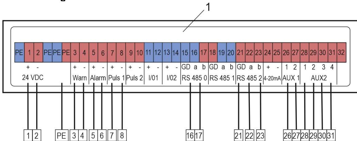
1 Klemmenbelegung
