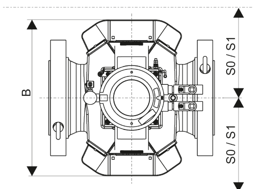
Draufsicht:
