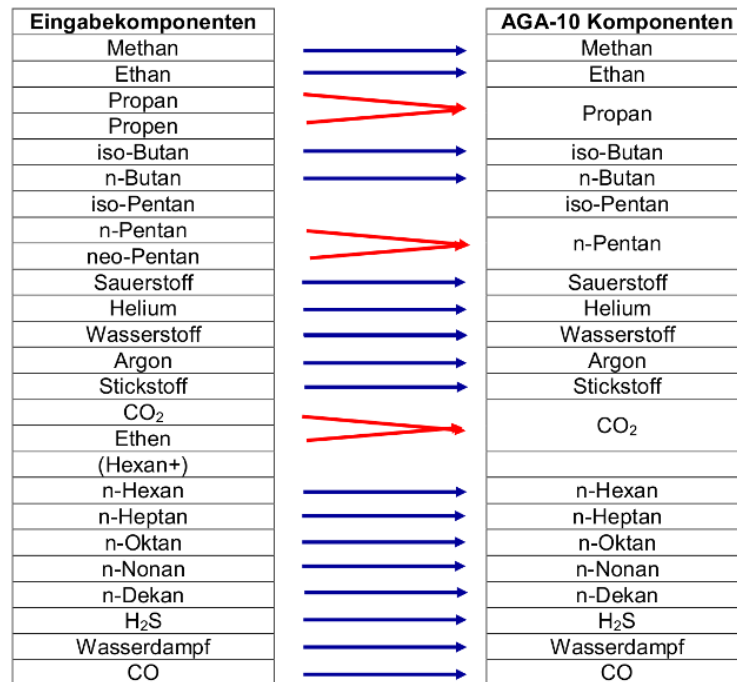
Abb. 4.8: Zuordnung der Gaskomponenten
