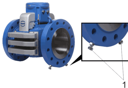
1 Stützschrauben
