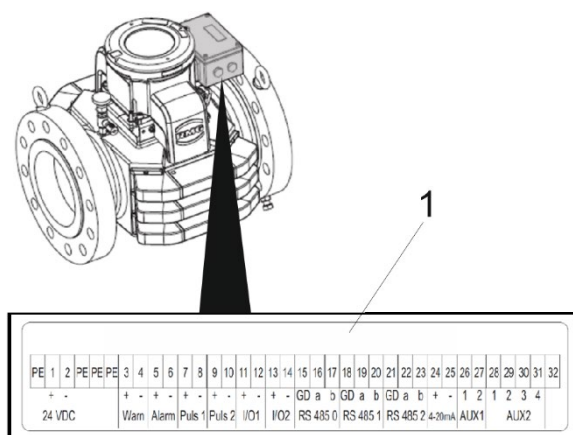
1 Klemmenbelegung
