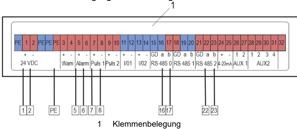
Abb. 8.7: Durchführung ½" mit 11 Adern Größe AWG 18 anschließen (Erlaubt max. 11; Killark Typ ENY-1TM).
