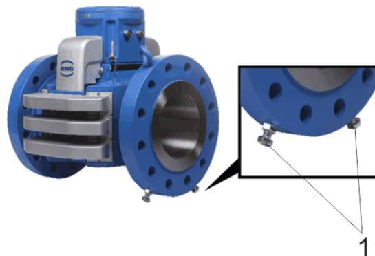
1 Stützschrauben mit Kontermuttern
