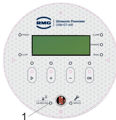
Abb. 10.6: Leuchtdiode prüfen
