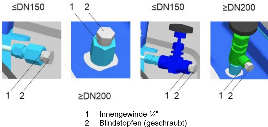
Abb. 8.44: Anschlussmöglichkeiten des Druckanschlusses mit Innengewinde
