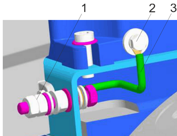
Abb. 2.2: Erdung – Ultraschallgaszähler DN100 (4") und DN150 (6")
