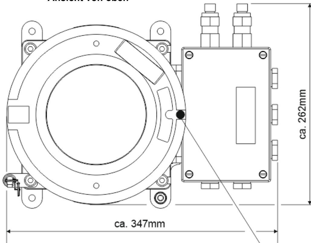
Plombe
