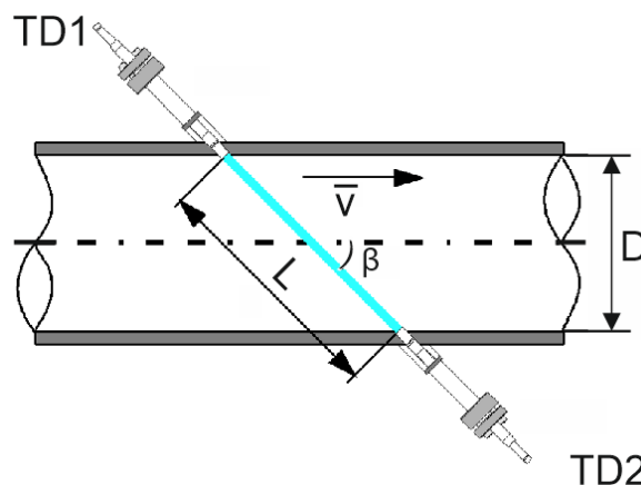
Abb. 4.1: Messung am Pfad
