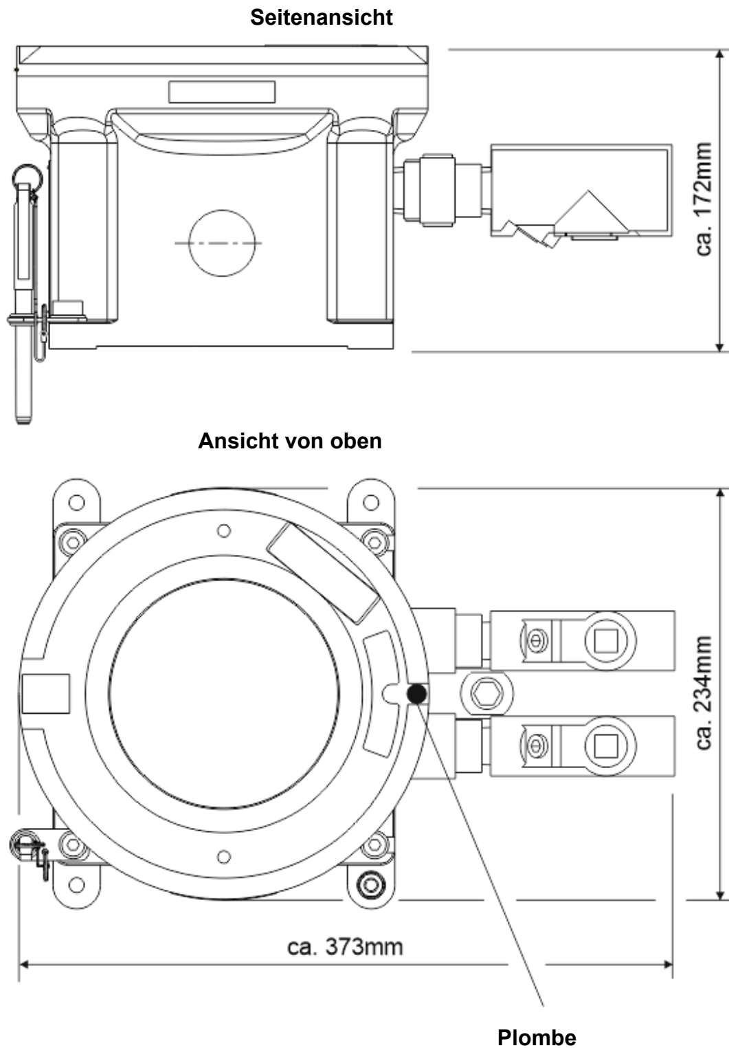
Abb. 13.10: Plombenplan gemäß NEC
