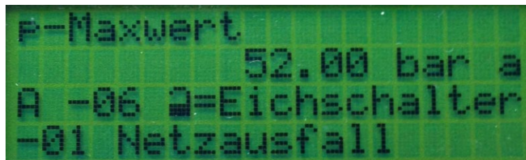
Abb. 3.3: Ultraschallelektronik Displayanzeige
