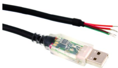
Abb. 8.38: TYP USB-RS485-WE-1800-BT 687-7834 (1,8 m) oder Typ USB-RS485-WE-5000-BT 730-0164 (5,0 m)
