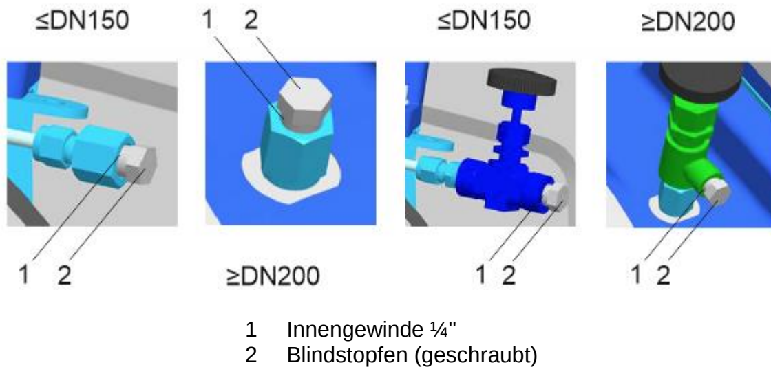
Abb. 8.33: Anschlussmöglichkeiten des Druckanschlusses mit Innengewinde
