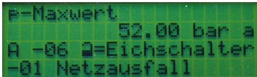
Abb. 3.3: Ultraschallelektronik Displayanzeige
