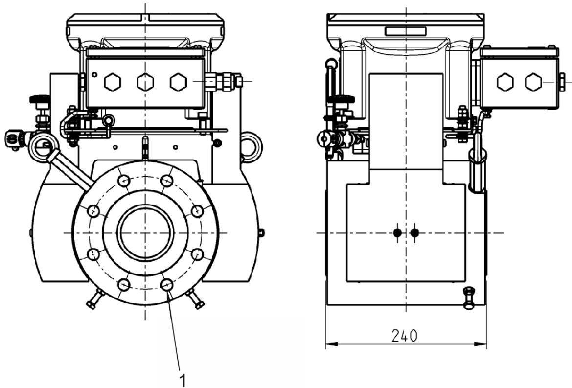
Abb. 13.6: Gewichte und Maße DN80
