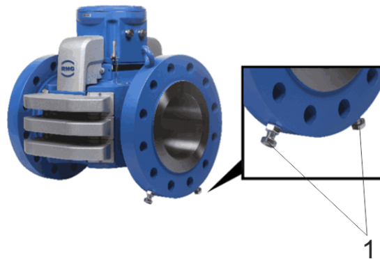
1 Stützschrauben
