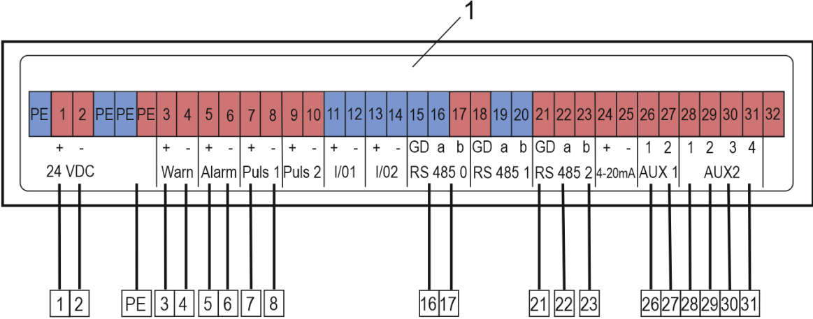
1 Klemmenbelegung
