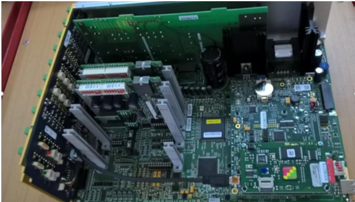
Abb. 8.14: Steckplatz für COM6 und 7 des ERZ 2000-NG
