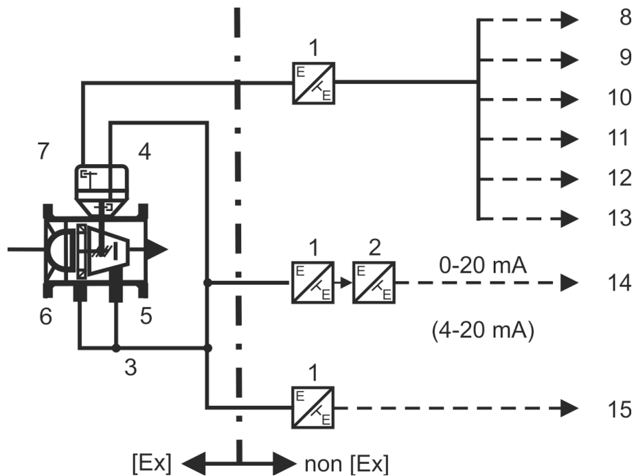
Abbildung 6: Anschlussmöglichkeiten am TRZ 03
