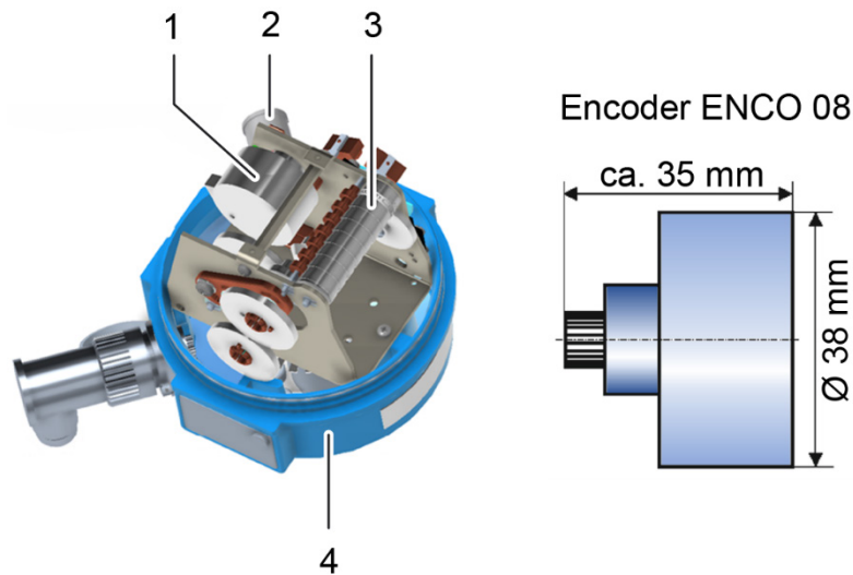
Abbildung 4: Encoder ENCO 08 im Zählwerkskopf Typ „F“ integriert
