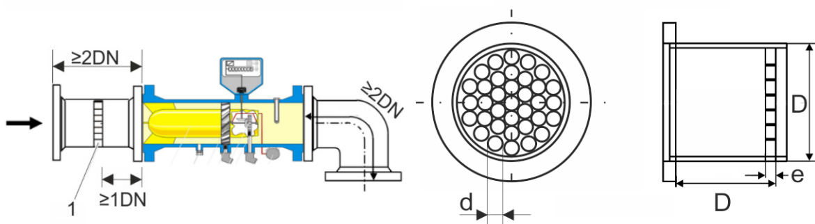
Lochplattengleichrichter LP-35
