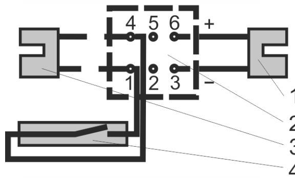
Abbildung 7: Steckerbelegung für den HF 1 Impulsgeber
