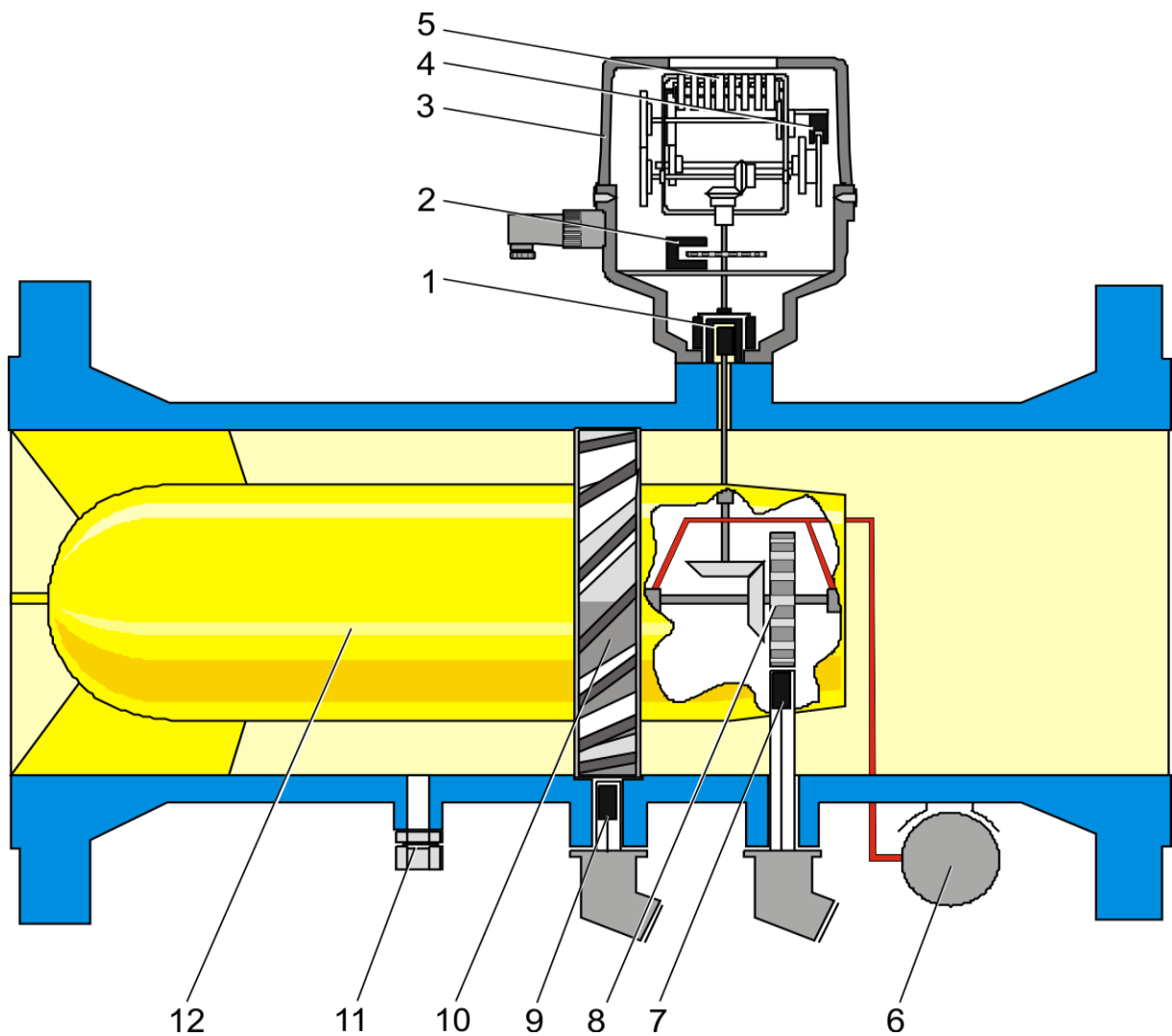
Abbildung 9: Schnittzeichnung Turbinenradgaszähler
