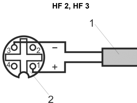
Abbildung 8: Steckerbelegung für den HF 2/3 Impulsgeber
