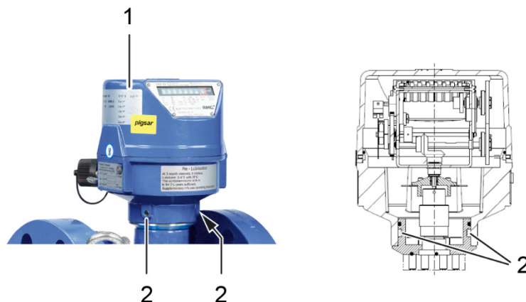
Abbildung 3: Zählwerkskopf Typ „F“
