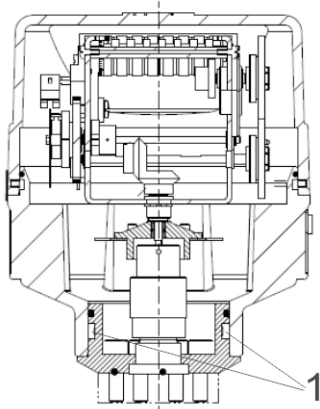
Abbildung 3: Zählwerkskopf Typ „F“
