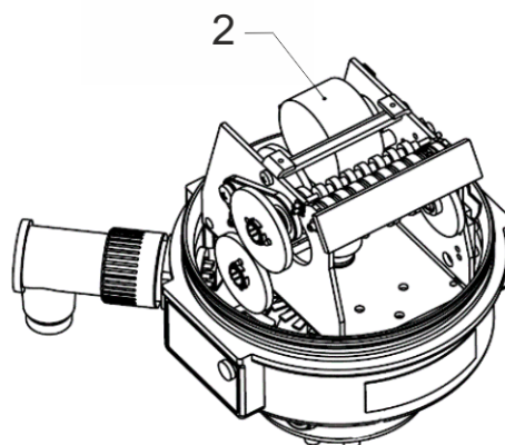
Abbildung 3: Zählwerkskopf Typ „F“
