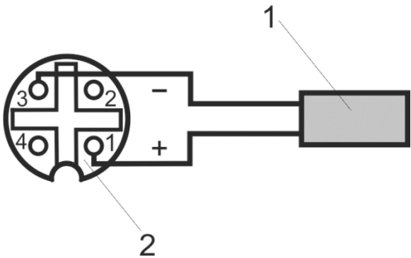
Abbildung 11: Steckerbelegung für den HF 2/3 Impulsgeber
