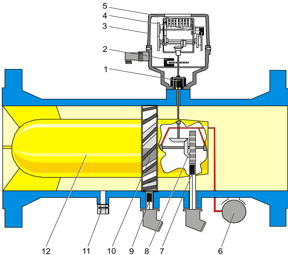
Abbildung 12: Schnittzeichnung Turbinenradgaszähler
