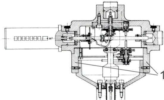
Abbildung 6: Zählwerkskopf Typ „D“
