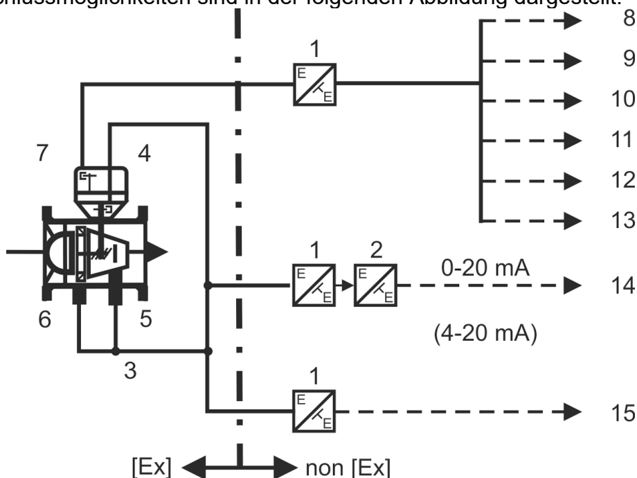
Abbildung 9: Anschlussmöglichkeiten am TRZ 03
