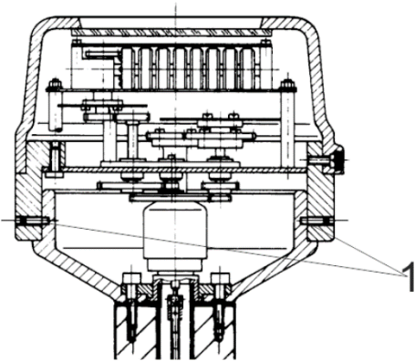
Abbildung 5: Zählwerkskopf Typ „A“
