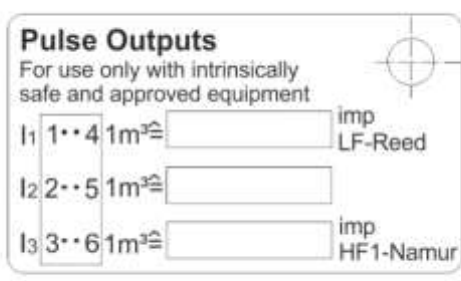
Emettitore di impulsi incorporato Testina di misura tipo „A“, „D“ e „F“ Solo per apparecchi con circuito elettrico a sicurezza intrinseca omologato
