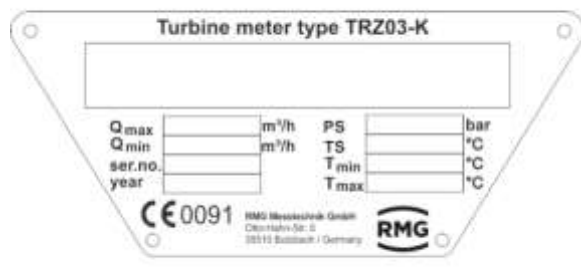
Targa principale contatori volumetrici con testina di misura tipo „F“
