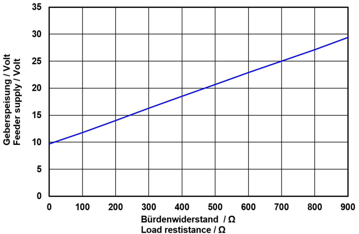
Bürde in Abhängigkeit Geberspeisung Load depending on feeder supply
