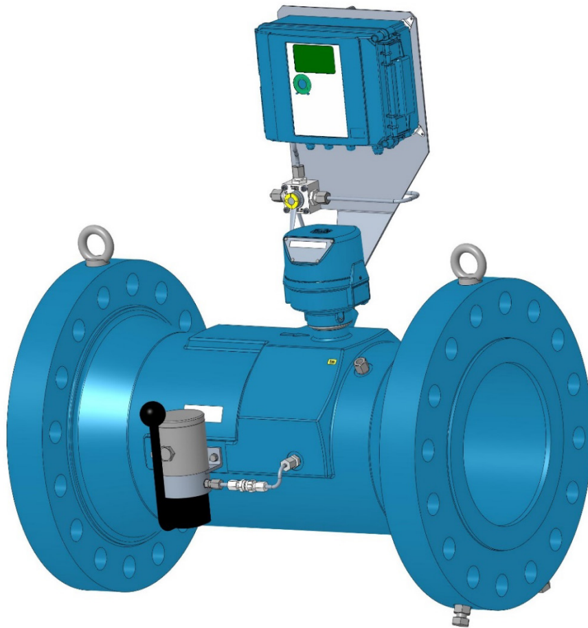
Abb. 8: Installation des Primus 400 am RMG Turbinengaszähler
