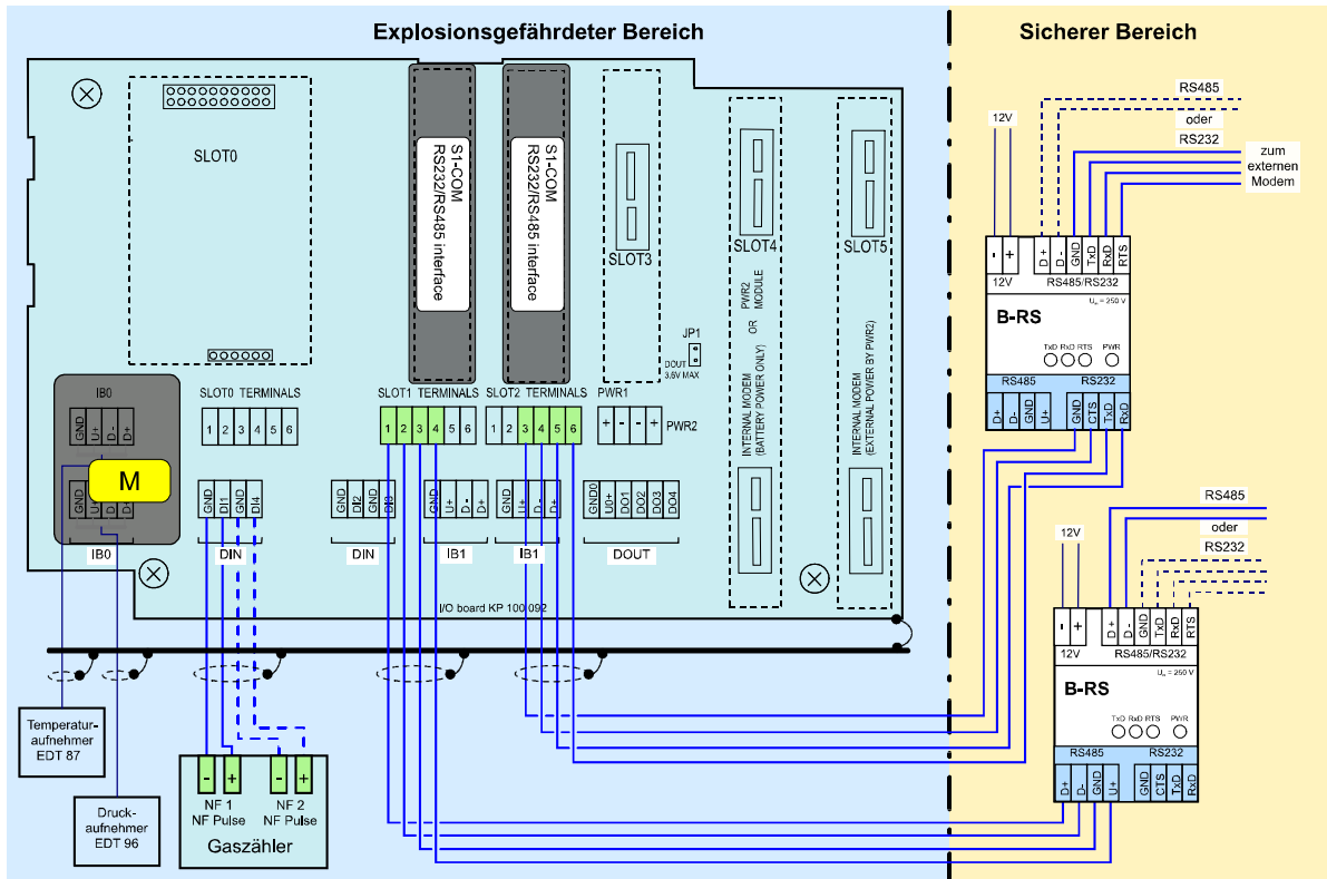
Abb. 24: Primus 400, Kommunikation über zwei unabhängige Schnittstellen RS232/RS485
