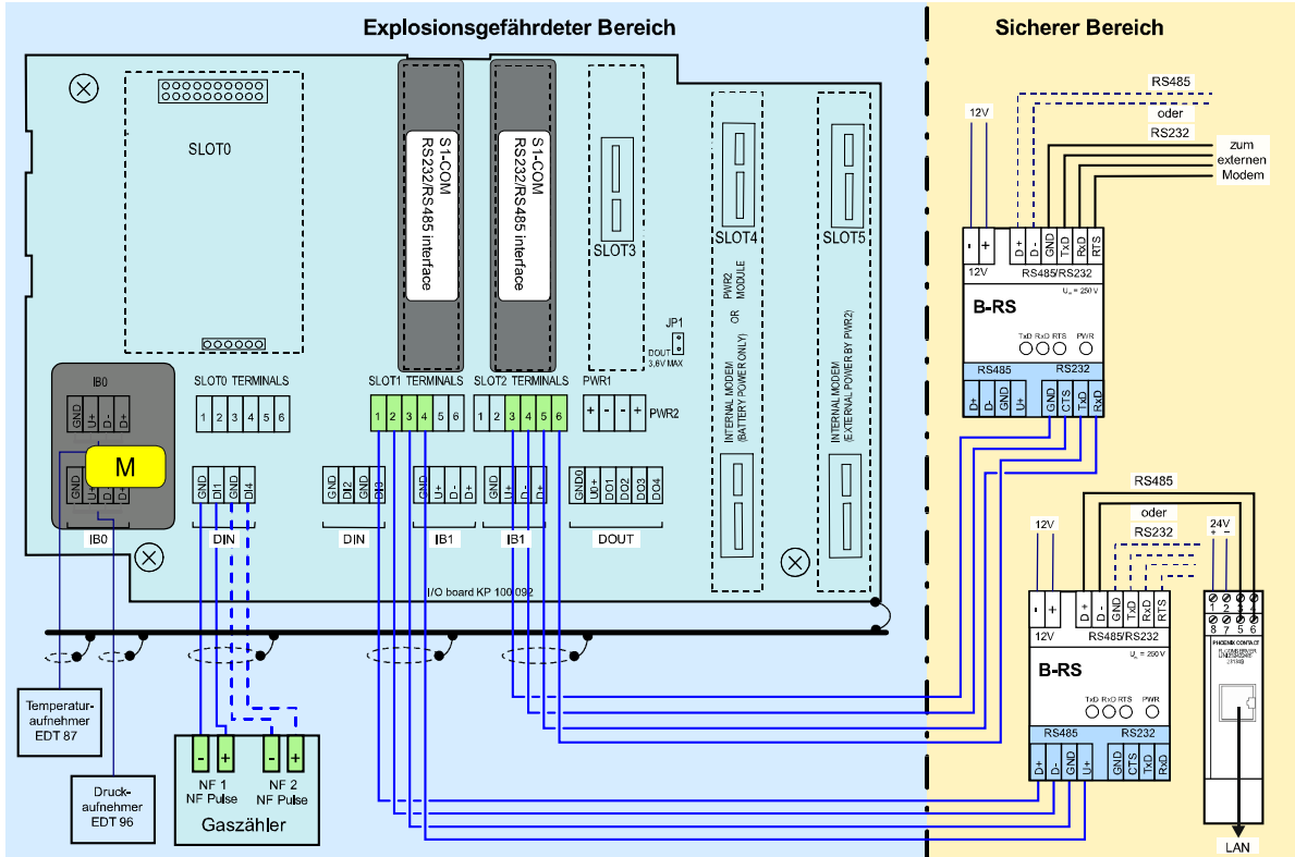
Abb. 25: Primus 400, Anschluss an RS232 sowie an LAN über RS485 und Comserver
