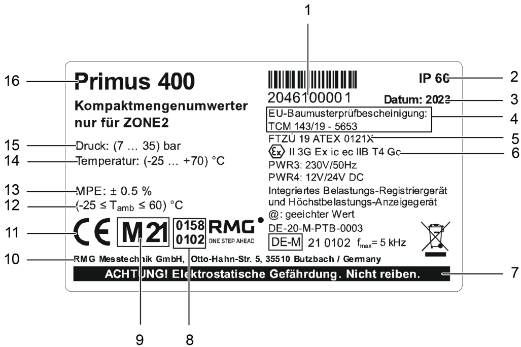
Abb. 76: Typenschild Primus 400 nur für Zone 2 (exemplarisch)
