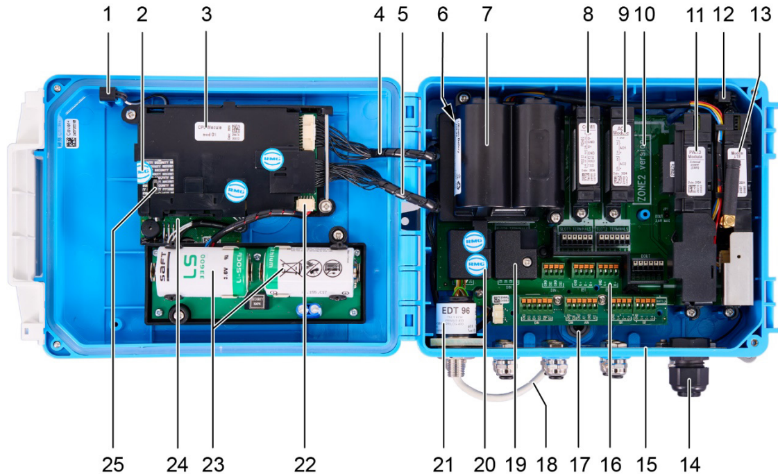
Abb. 46: Hauptkomponenten des Primus 400
