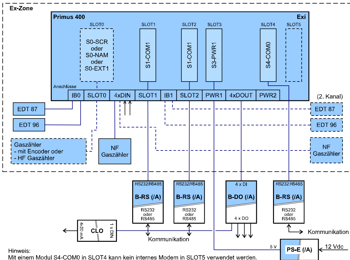
Abb. 75: Primus 400, Verwendungsbeispiel 2 für externe Module
