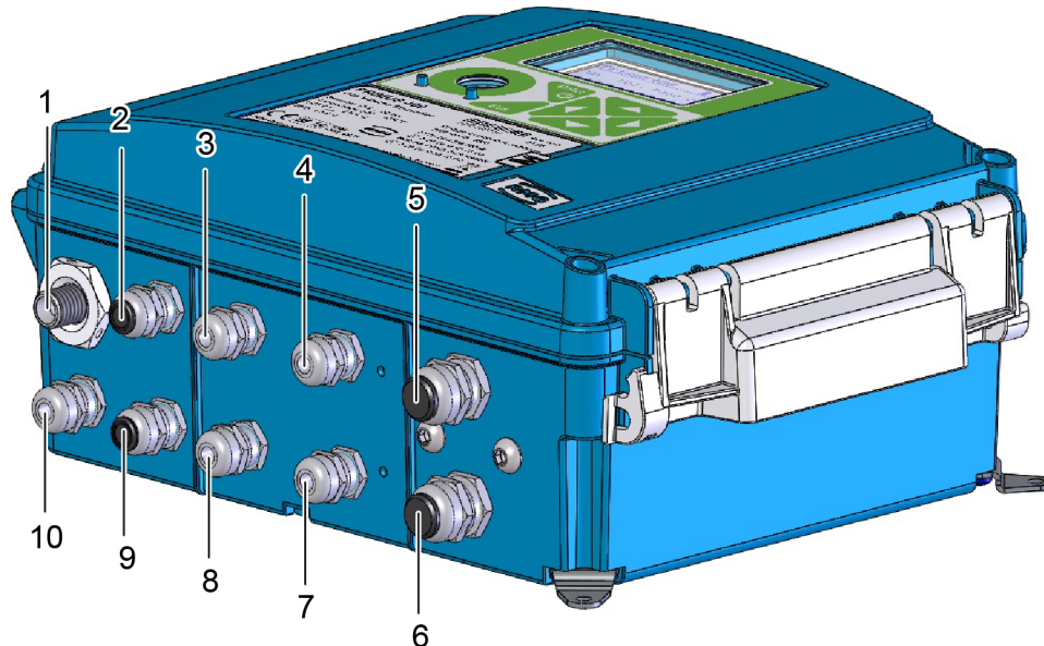
Abb. 78: Anordnung der Kabelverschraubungen
