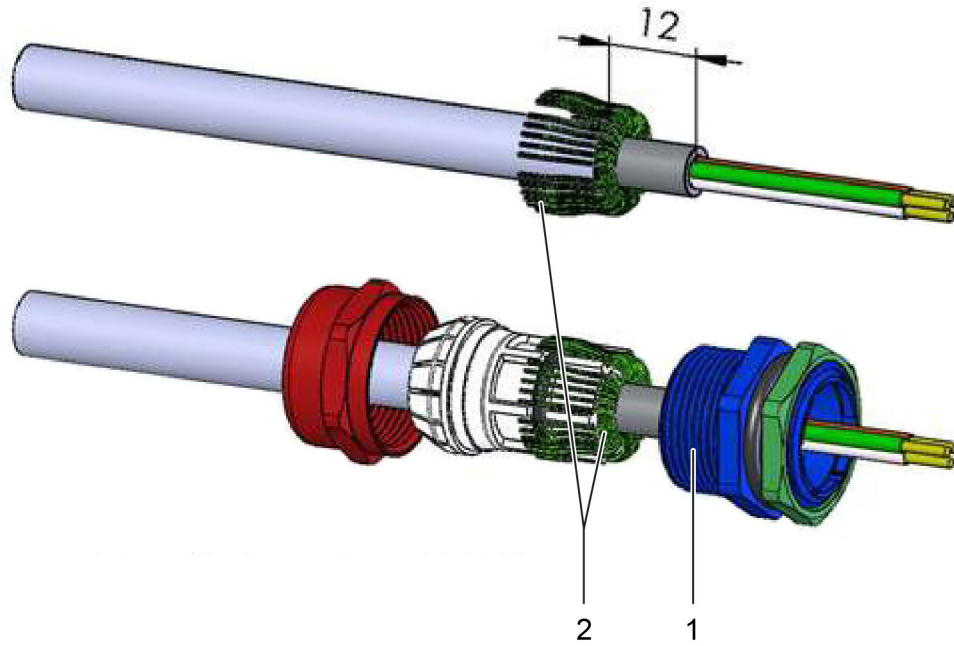
Abb. 11: Verbindung der Kabelabschirmungen in den Kabelverschraubungen
