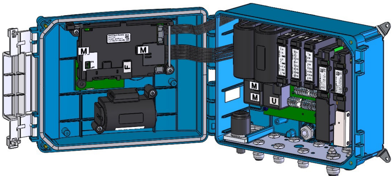
Abb. 2: Innere Sicherheitsmarken des Primus 400
