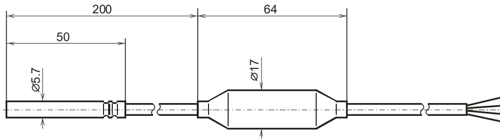
Abb. 62: Sensorabmessungen
