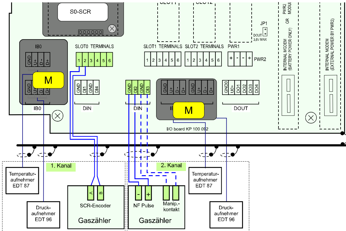
Abb. 17: Anschließen des Gaszählers mit SCR-Encoder am Primus 400
