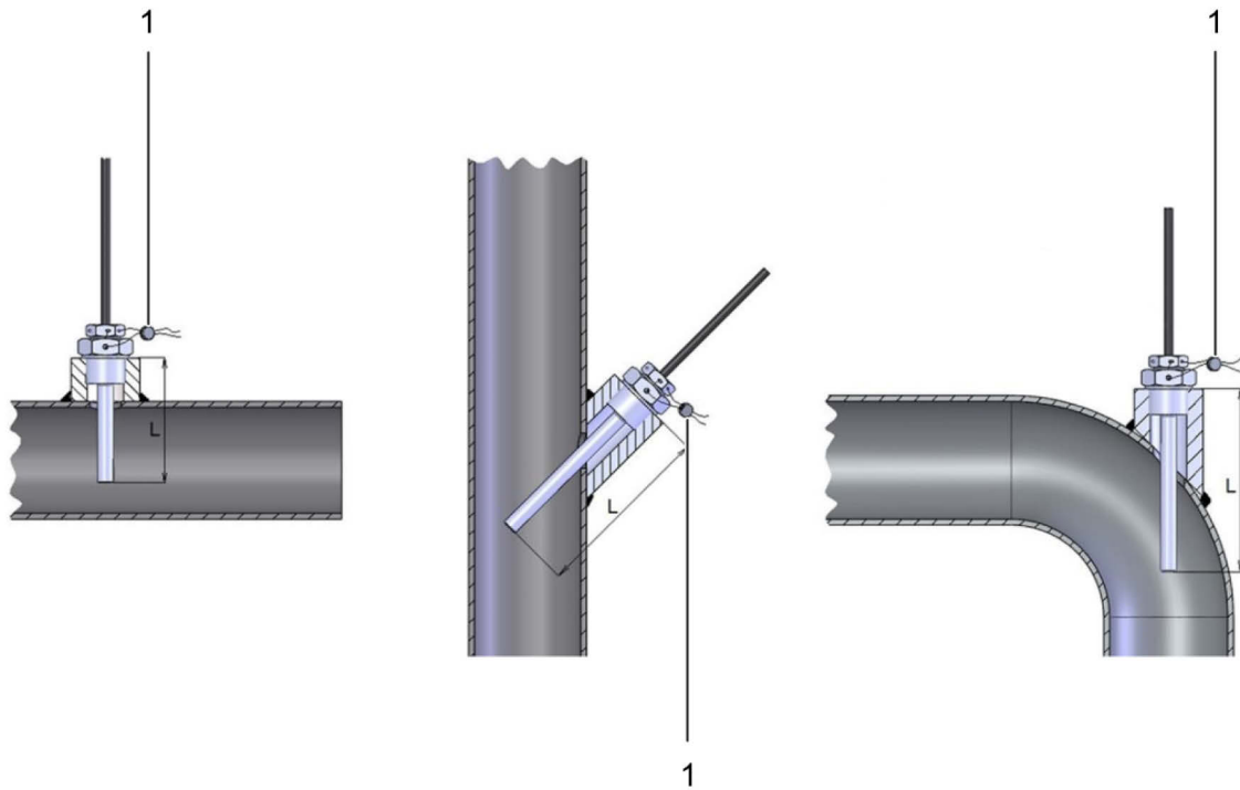
Abb. 9: Montage des Temperatursensors an der Gasleitung
