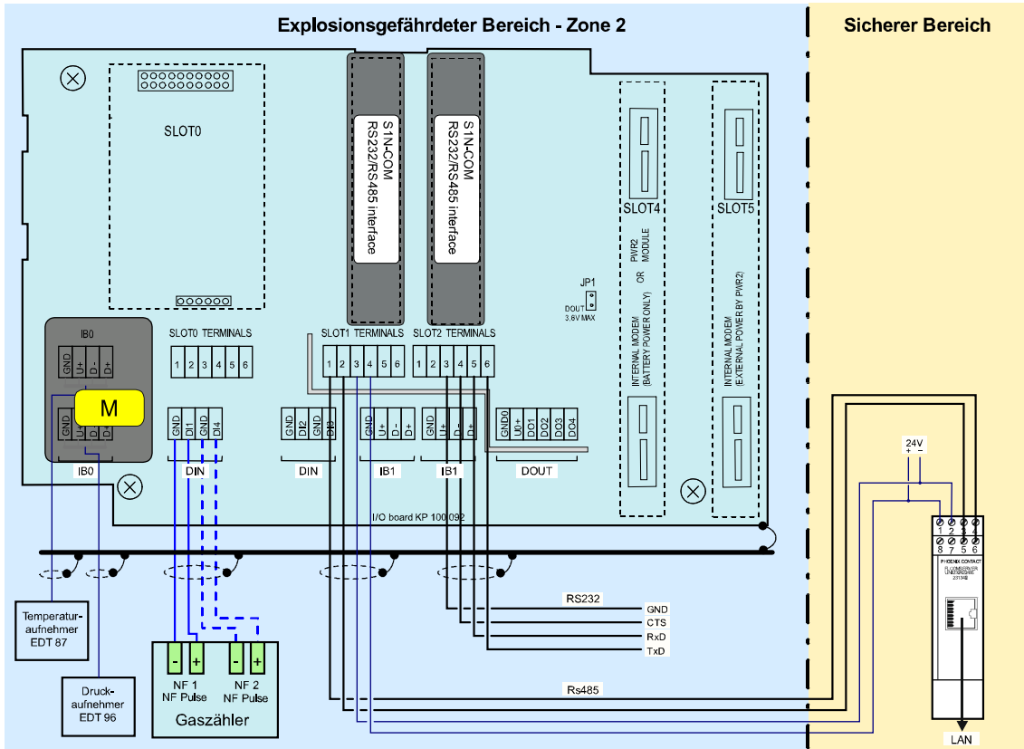
Abb. 81: Primus 400, Anschluss an LAN über RS485 und Comserver
