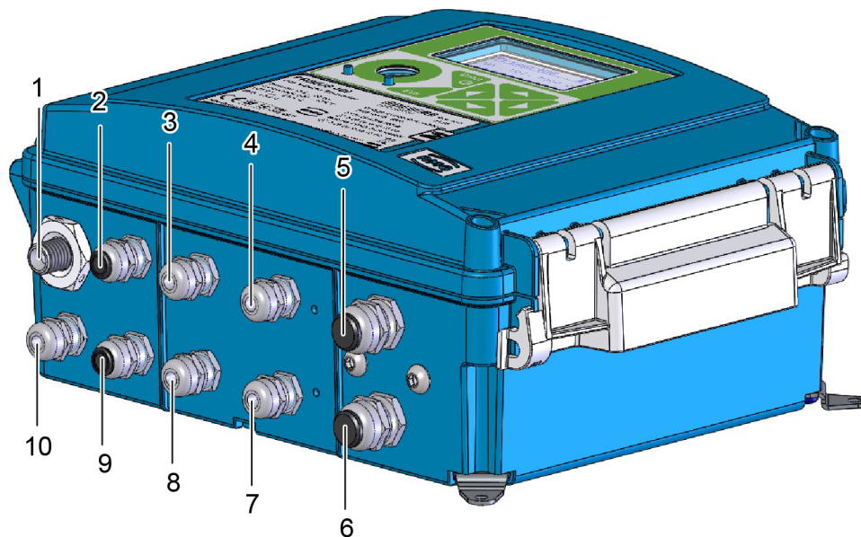
Abb. 12: Anordnung der Kabelverschraubungen
