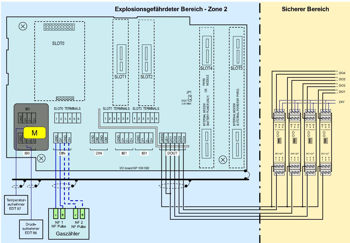
Abb. 80: Anschließen der Digitalausgänge über die Trennbarrieren IM1-12-T (Primus 400)
