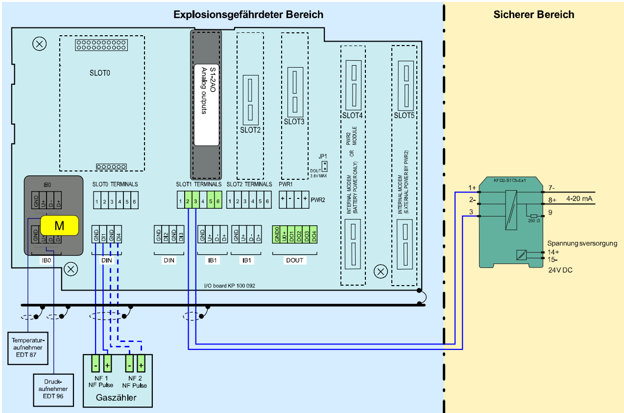
Abb. 19: Anschließen der Analogausgänge über die Trennbarriere KFD2-STC5-Ex1 (Primus 400)
