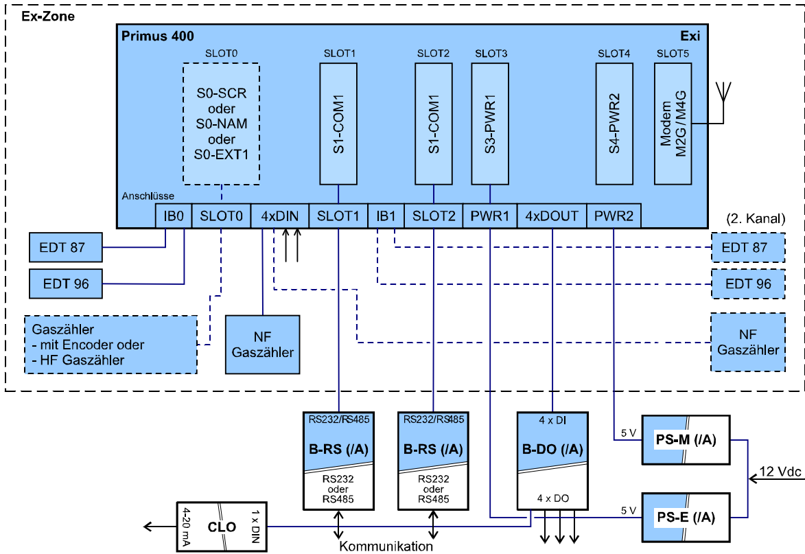
Abb. 74: Primus 400, Verwendungsbeispiel 1 für externe Module
