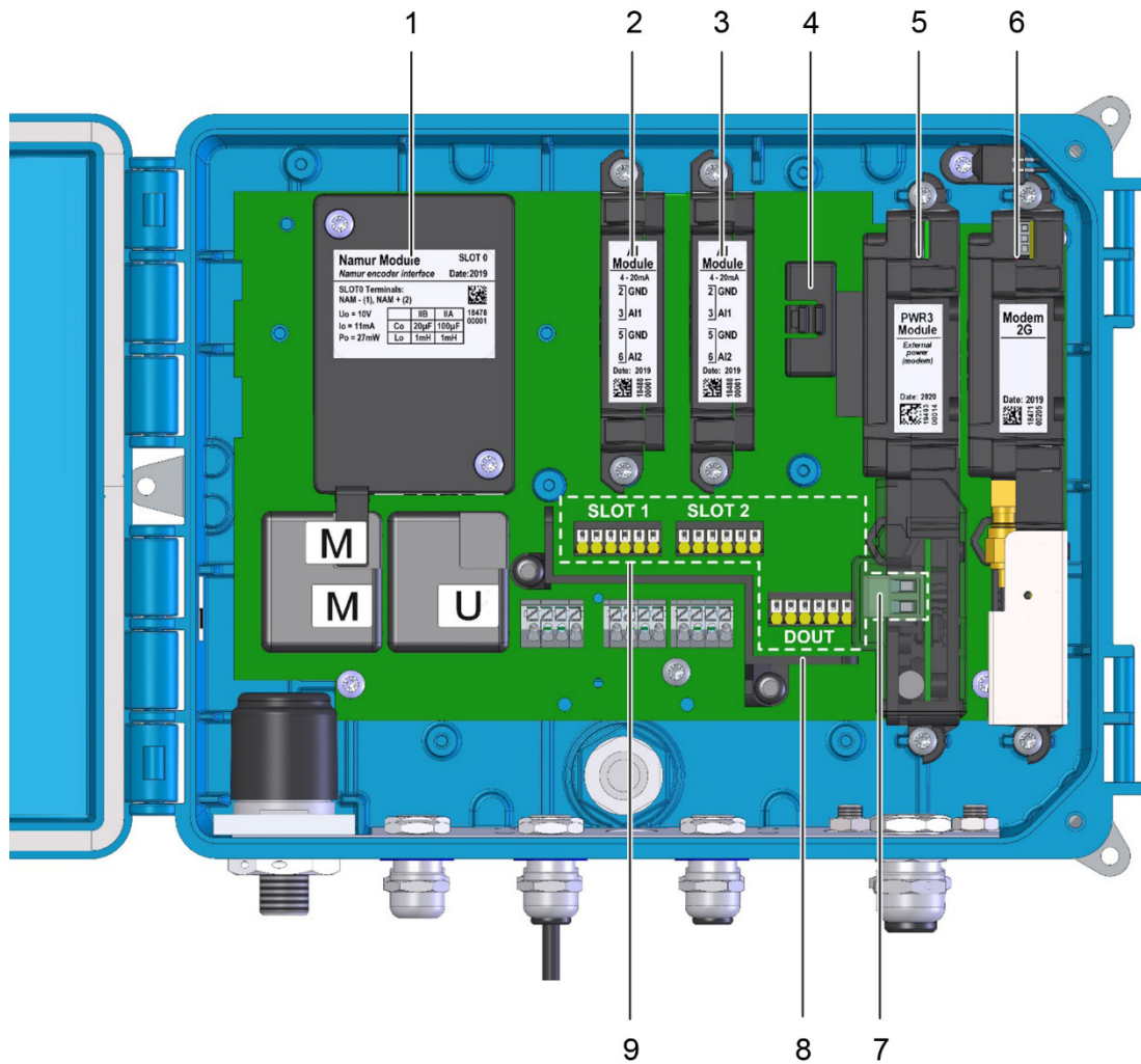
Abb. 77: Klemmen mit Schutz „ec“
