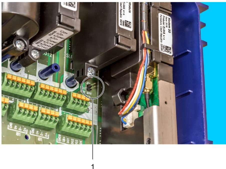
Abb. 58: Installation der Brücke JP1 auf der E/A-Karte
