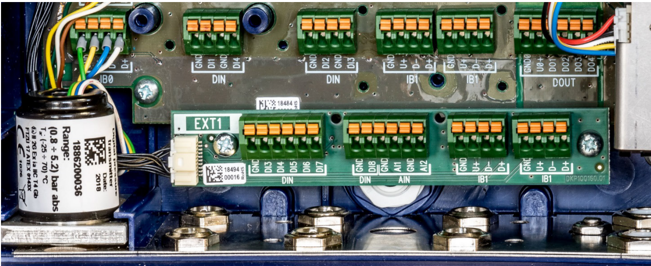
Abb. 65: Zusatzanschlusskarte EXT1-T für das Modul S0-EXT1
