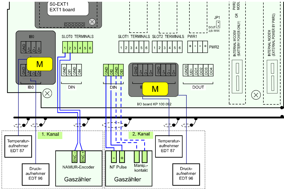
Abb. 16: Anschließen des Gaszählers mit NAMUR-Encoder am Primus 400
