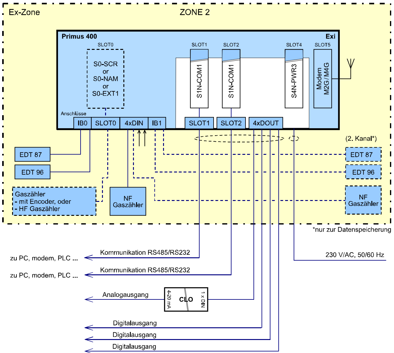
Abb. 83: Blockschaltbild, Primus 400 für Zone 2 mit ext. 230V Spannungsversorgung
