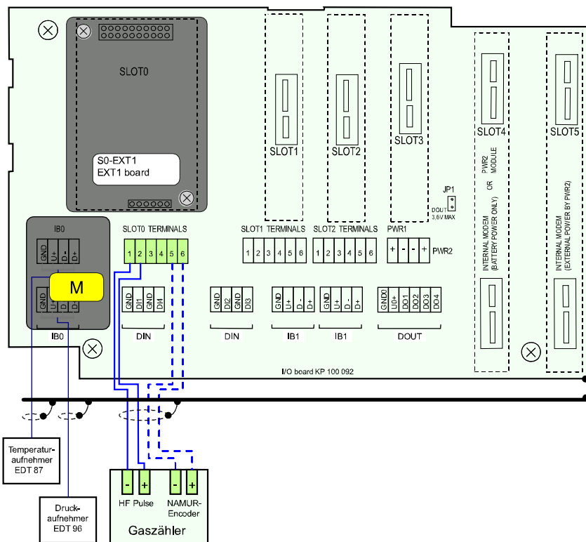
Abb. 15: Anschließen der HF-Gaszähler (optional mit Encoder) am Primus 400
