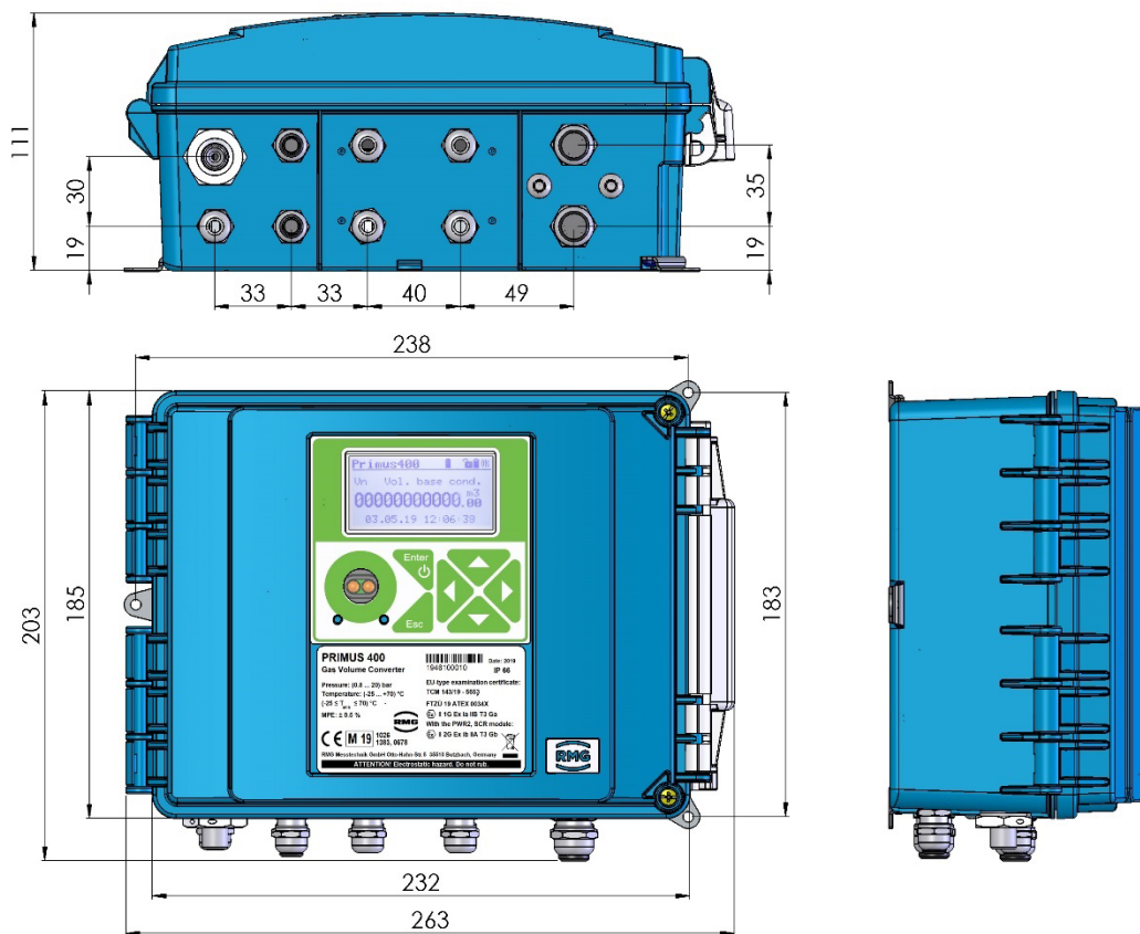
Abb. 1: Primus 400 Geräteabmessungen
