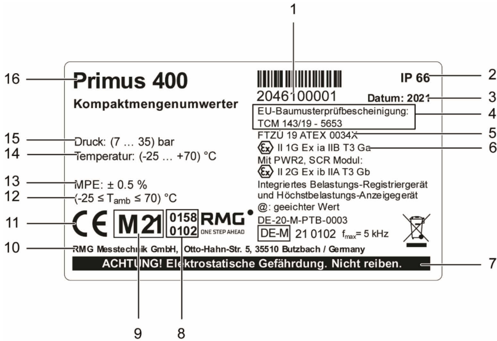
Abb. 4: Typenschild (exemplarisch)
