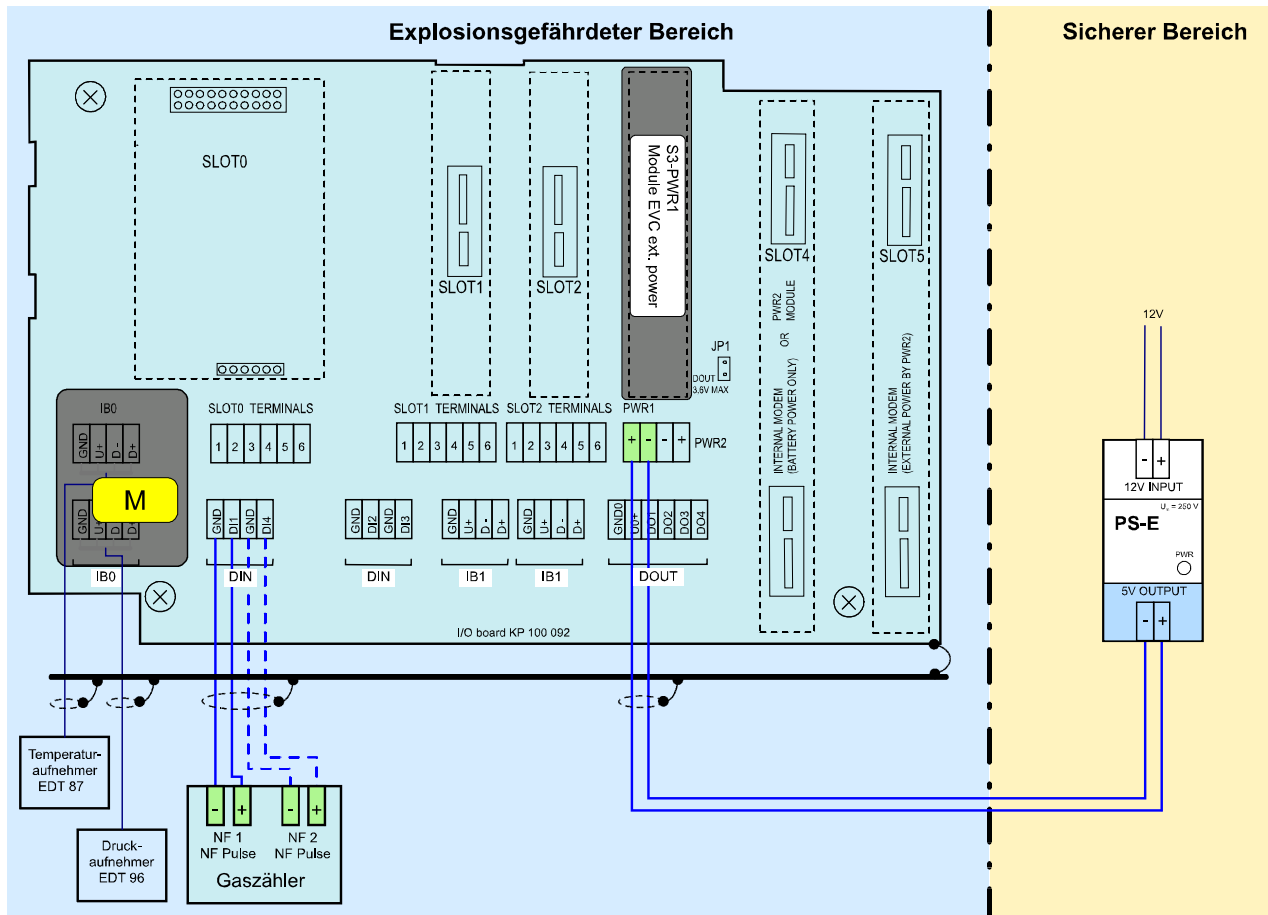
Abb. 21: Anschließen der externen Spannungsversorgung des Mengenumwerters
