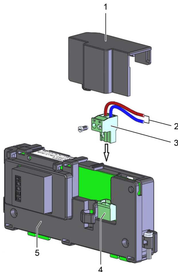
Abb. 79: Anschluss der externen Spannungsversorgung
