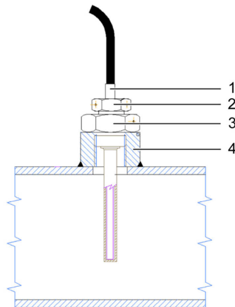
Abb. 10: Montage des Temperatursensors mit einem geraden Schweißnippel
