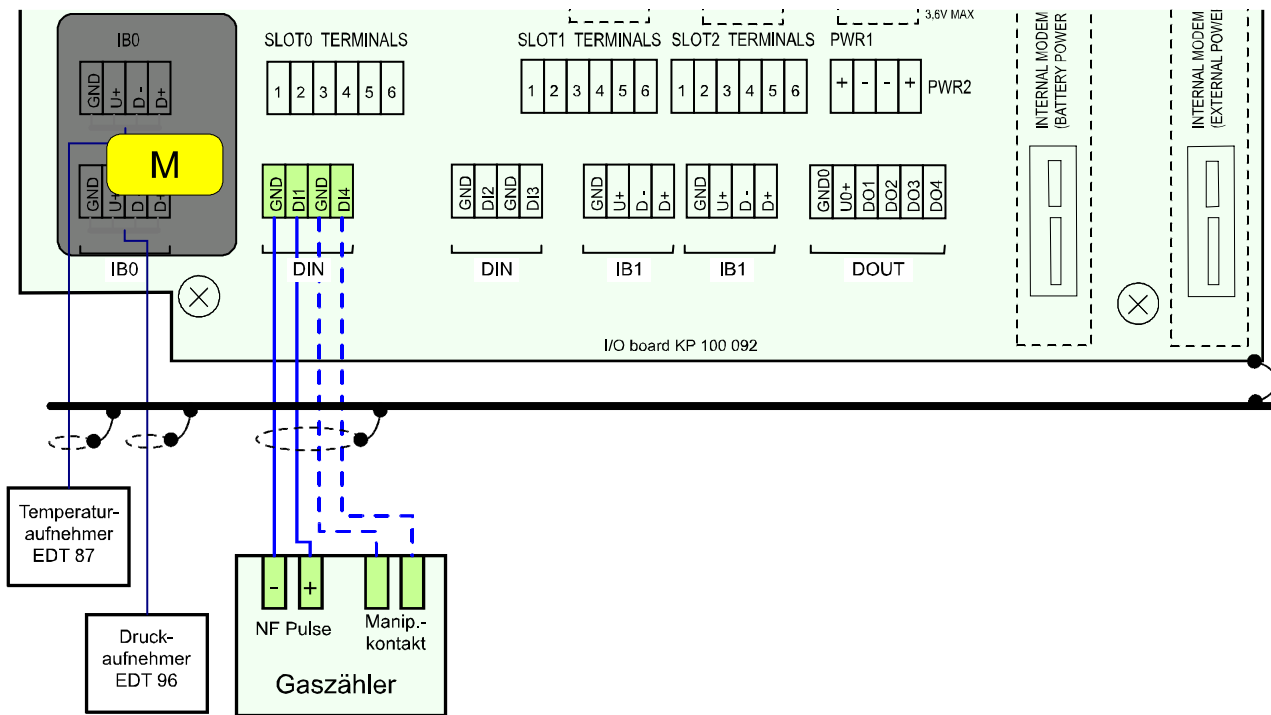
Abb. 13: Anschließen des NF-Gaszählers am Primus 400 (Einkanal)
