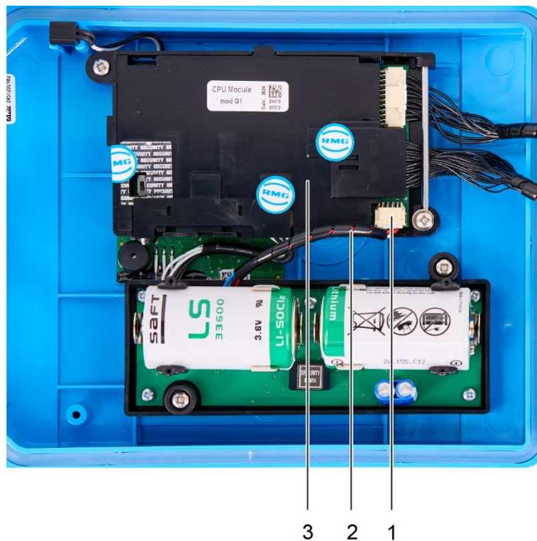
Abb. 26: Anschließen der Gerätebatterie
