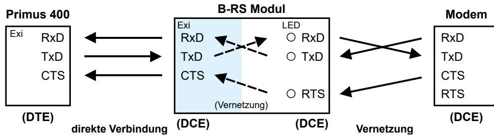
Abb. 66: Anschlussprinzip mit PC und externem Modem über das Modul B-RS
