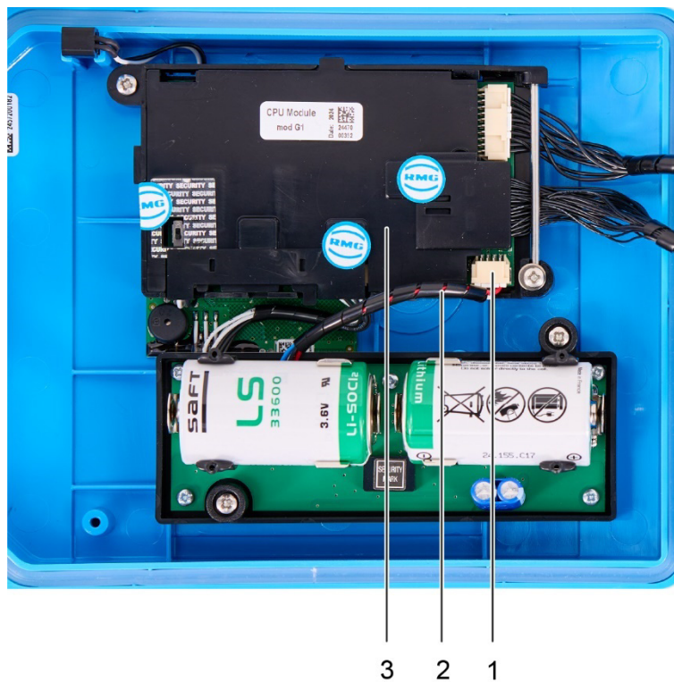
Abb. 56: Hauptbatterie
