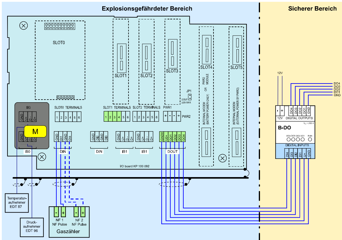
Abb. 18: Anschließen der Digitalausgänge über die Trennbarriere B-DO (Primus 400)
