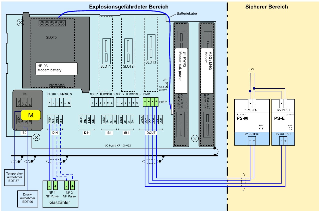
Abb. 23: Externe Spannungsversorgung des Mengenumwerters und des internen Modems
