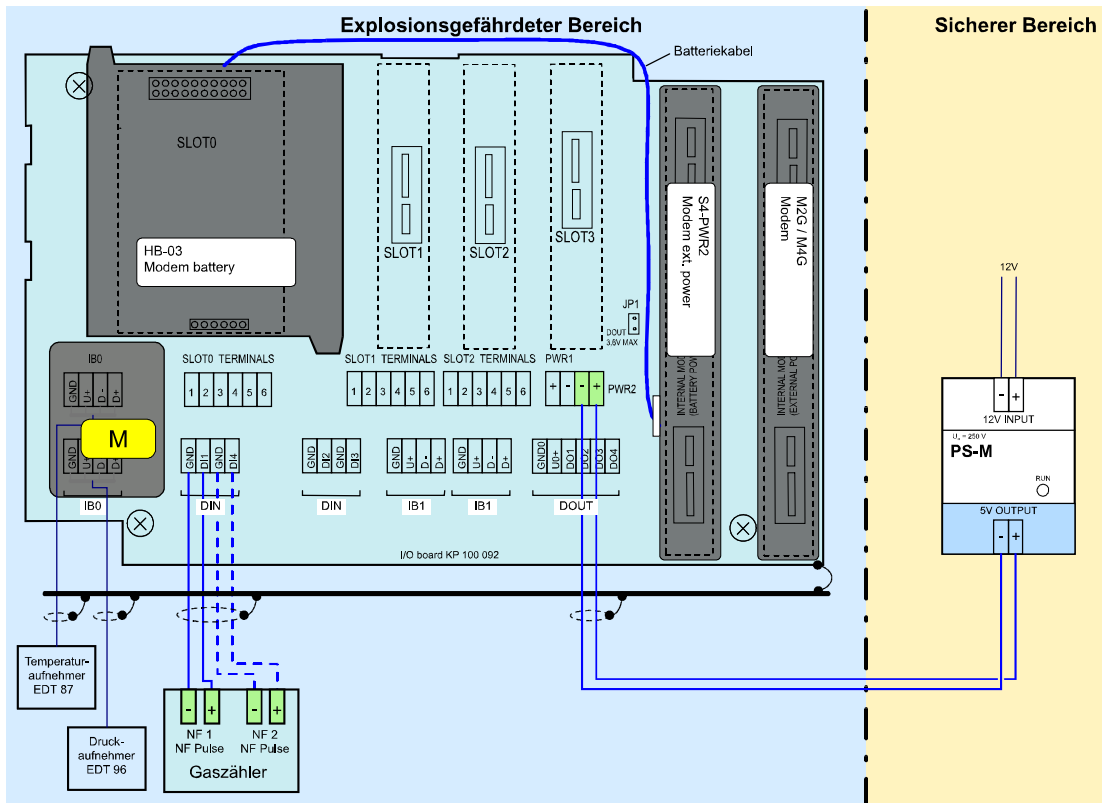
Abb. 22: Externe Spannungsversorgung PS-M für das interne Modem mit der Versorgung PS-M
