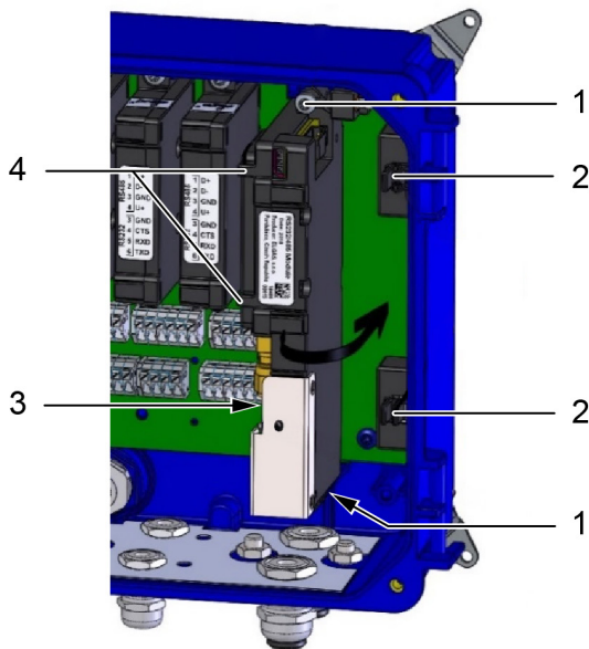
Abb. 53: Installieren ext. Spannungsversorgung Abb. 54: Demontieren der Anschlusskappen
