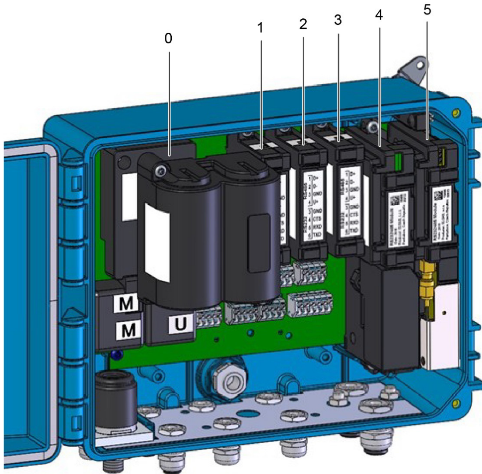
Abb. 48: Anordnung der Steckplätze (Slots) des Primus 400
