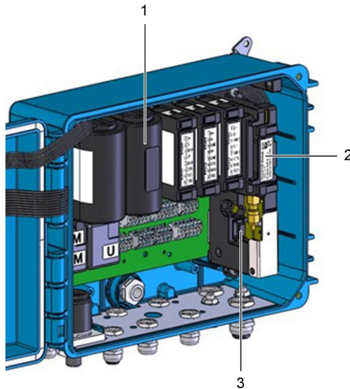
Abb. 27: Anschließen der Modembatterie für Primus 400
