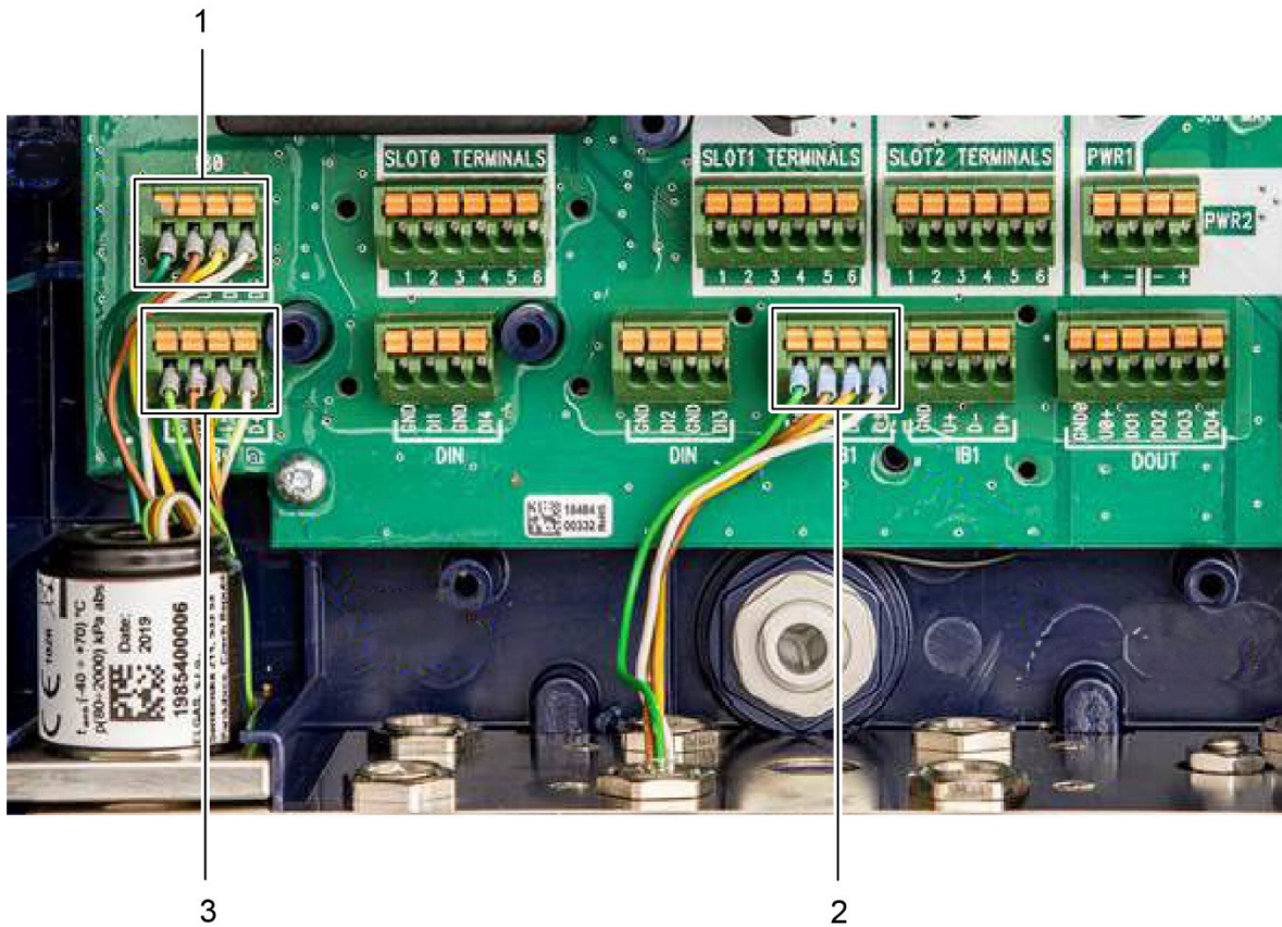
Abb. 20: Anschluss der Sensoren EDT 96 und EDT 87
