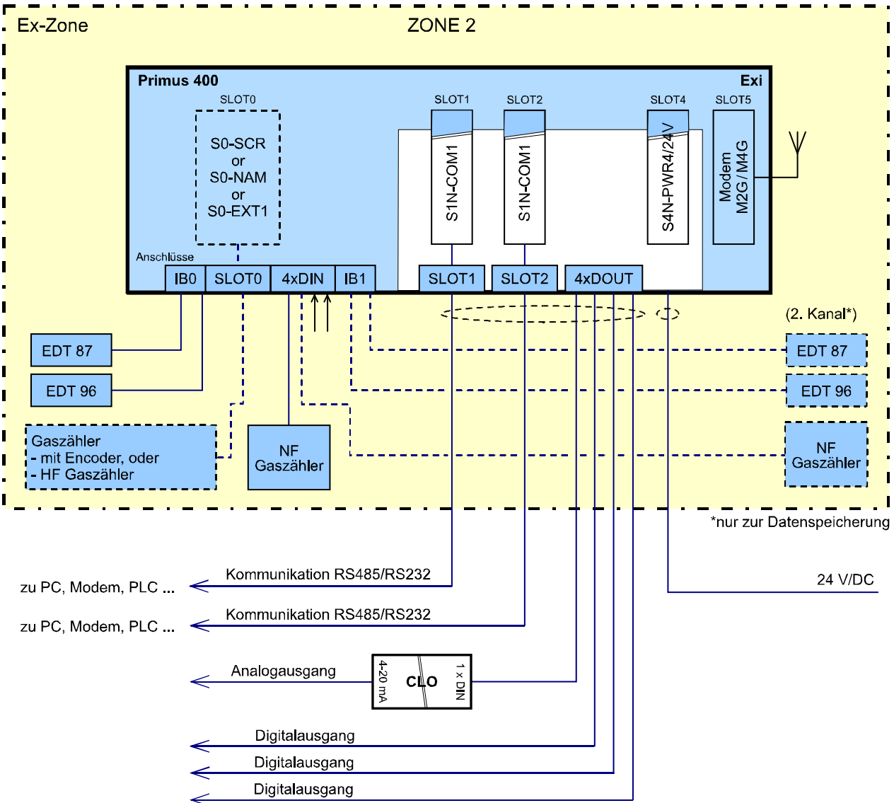
Abb. 82: Blockschaltbild, Primus 400 für Zone 2 mit ext. 24V Spannungsversorgung
