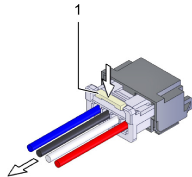
Abb. 52: Steckersperre lösen
