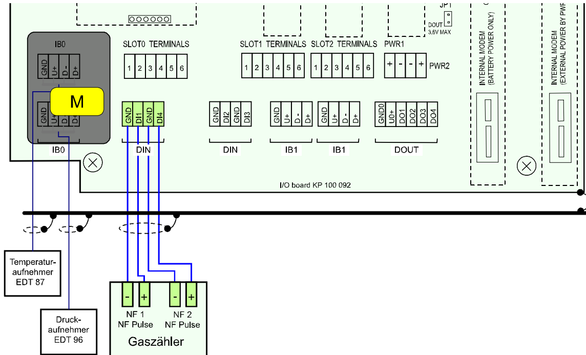
Abb. 14: Anschließen des NF-Gaszähler mit Erkennung der Drehrichtung am Primus 400
