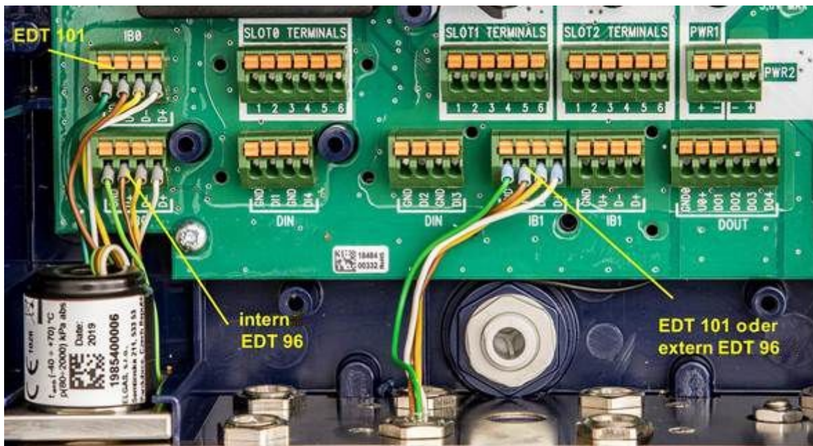
Abb. 18: Anschluss der Sensoren EDT 96 und EDT 101
