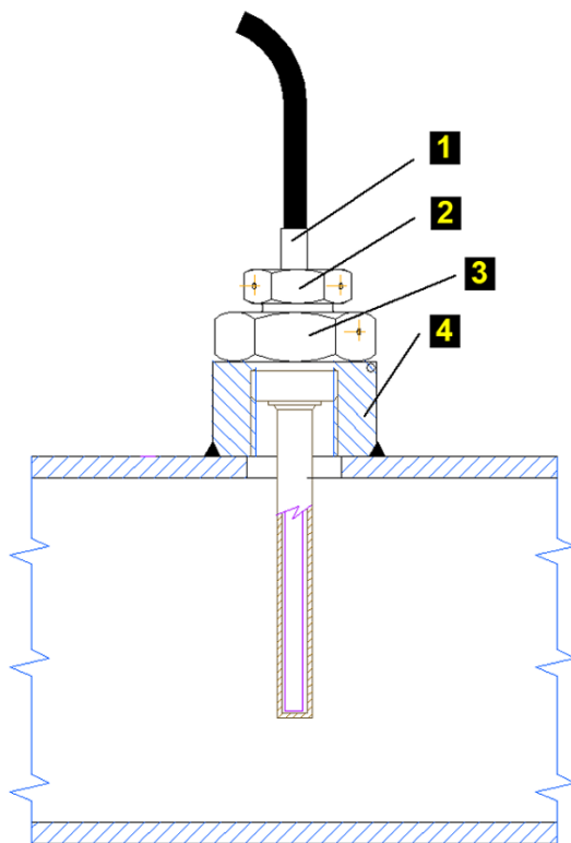
Abb. 9: Montage des Temperatursensors mit einem geraden Schweißnippel
