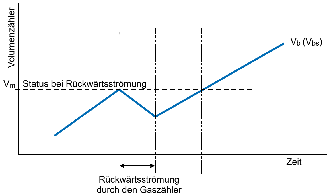
Abb. 43: Verarbeitung der Volumina bei umgekehrter Gaszählerdrehung
