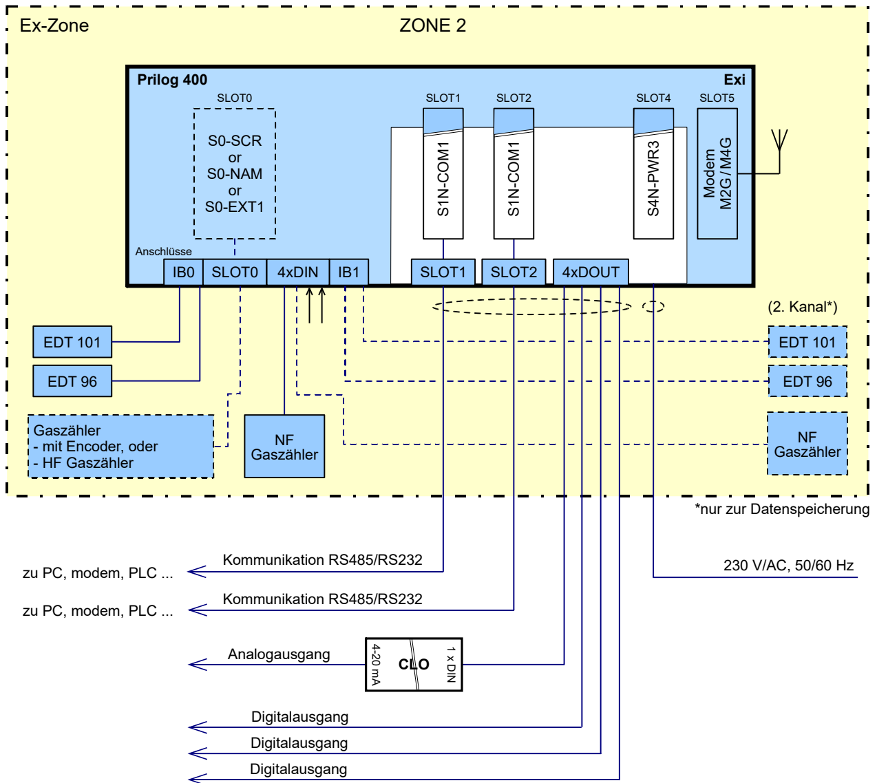
Abb. 61: Blockschaltbild, Prilog 400 für Zone 2 mit ext. 230V Spannungsversorgung
