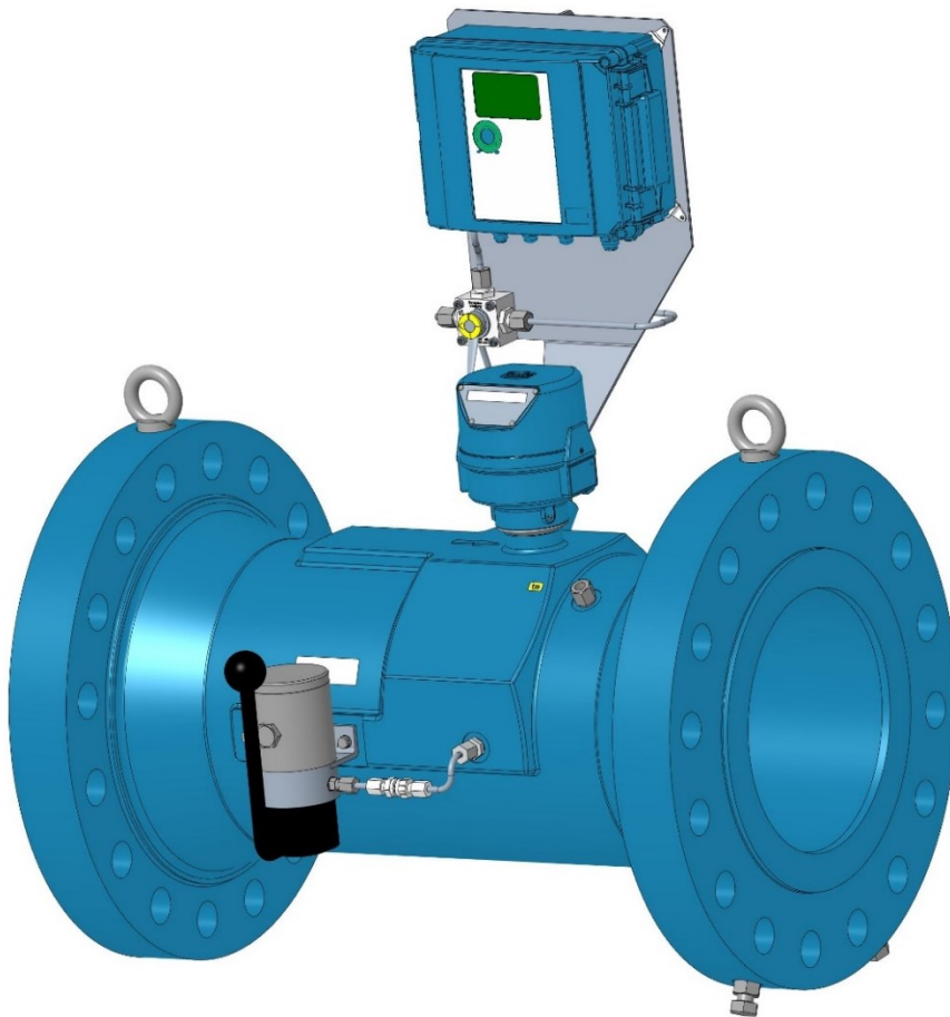
Abb. 7: Installation des Prilog 400 am RMG Turbinengaszähler
