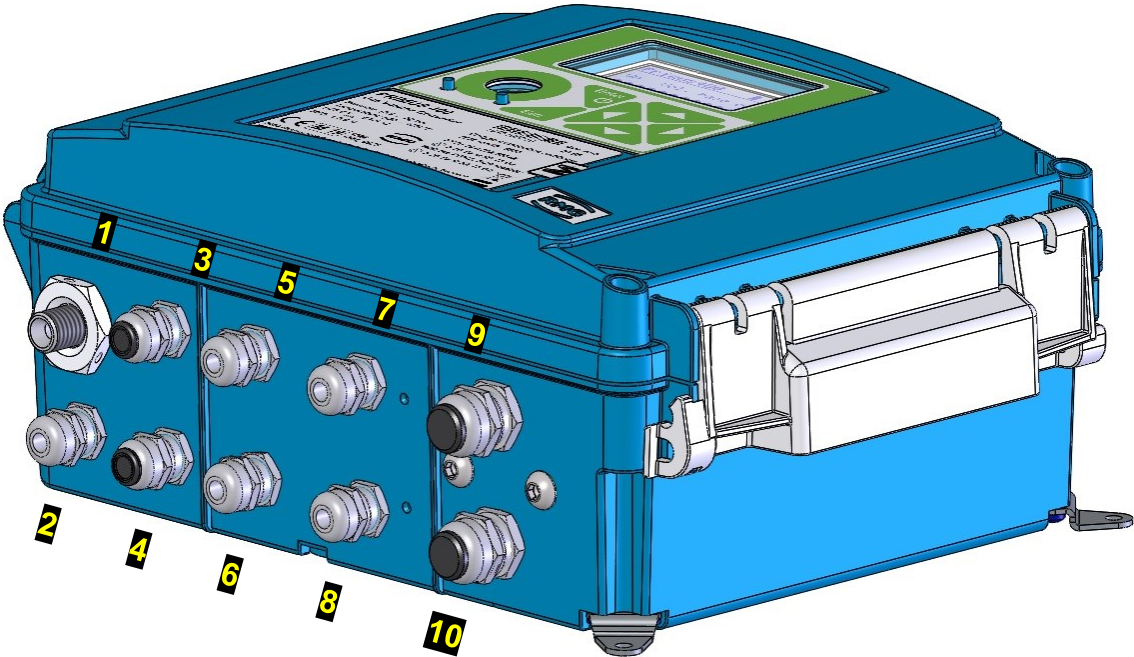
Abb. 11: Anordnung der Kabelverschraubungen
