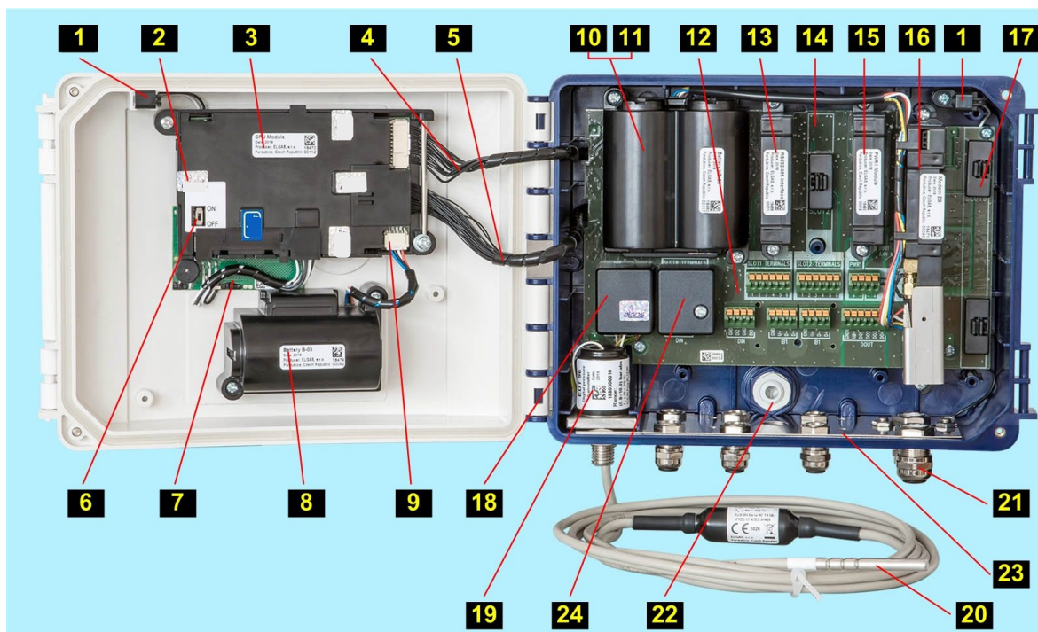
Abb. 35: Hauptkomponenten des Prilog 400
