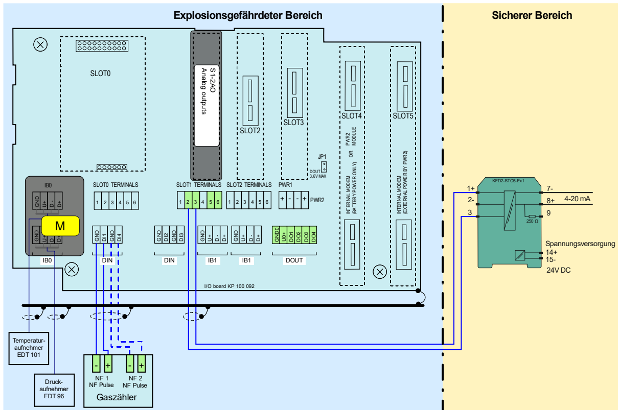
Abb. 17: Anschließen der Analogausgänge über die Trennbarriere KFD2-STC5-Ex1 (Prilog 400)
