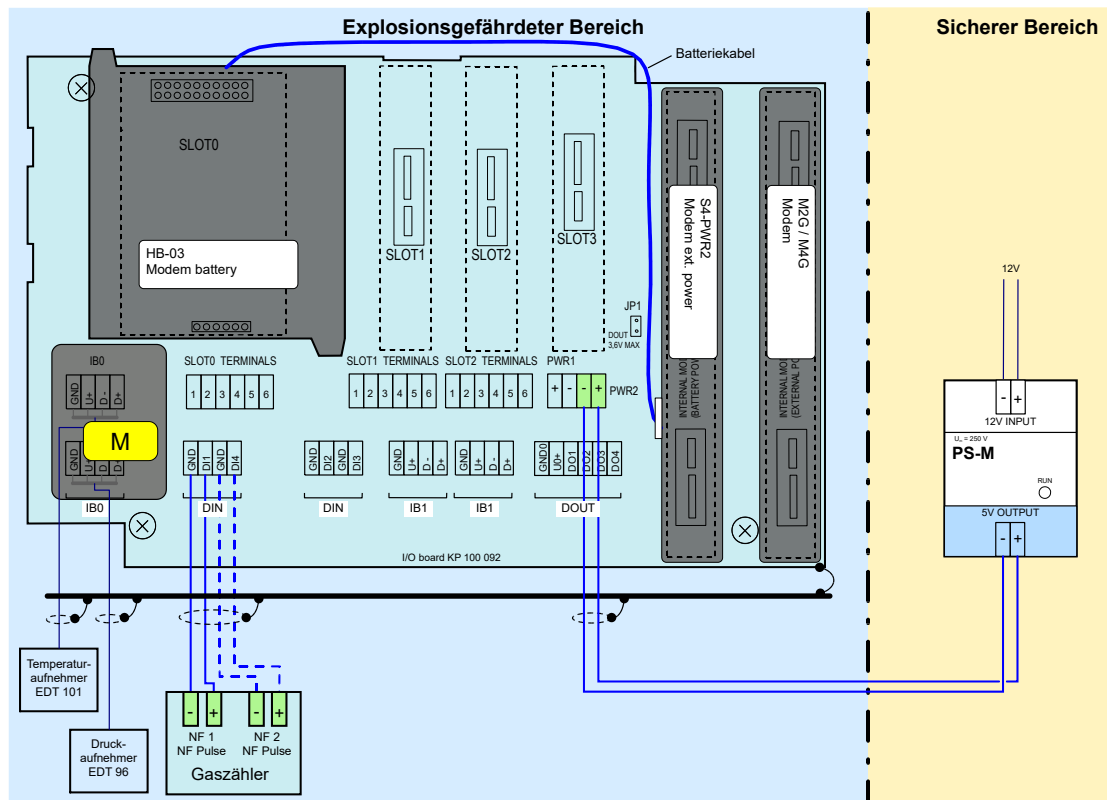
Abb. 20: Externe Spannungsversorgung PS-M für das interne Modem mit der Versorgung PS-M
