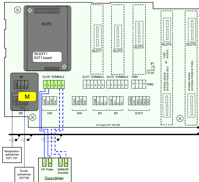
Abb. 13: Anschließen der HF-Gaszähler (optional mit Encoder) am Prilog 400
