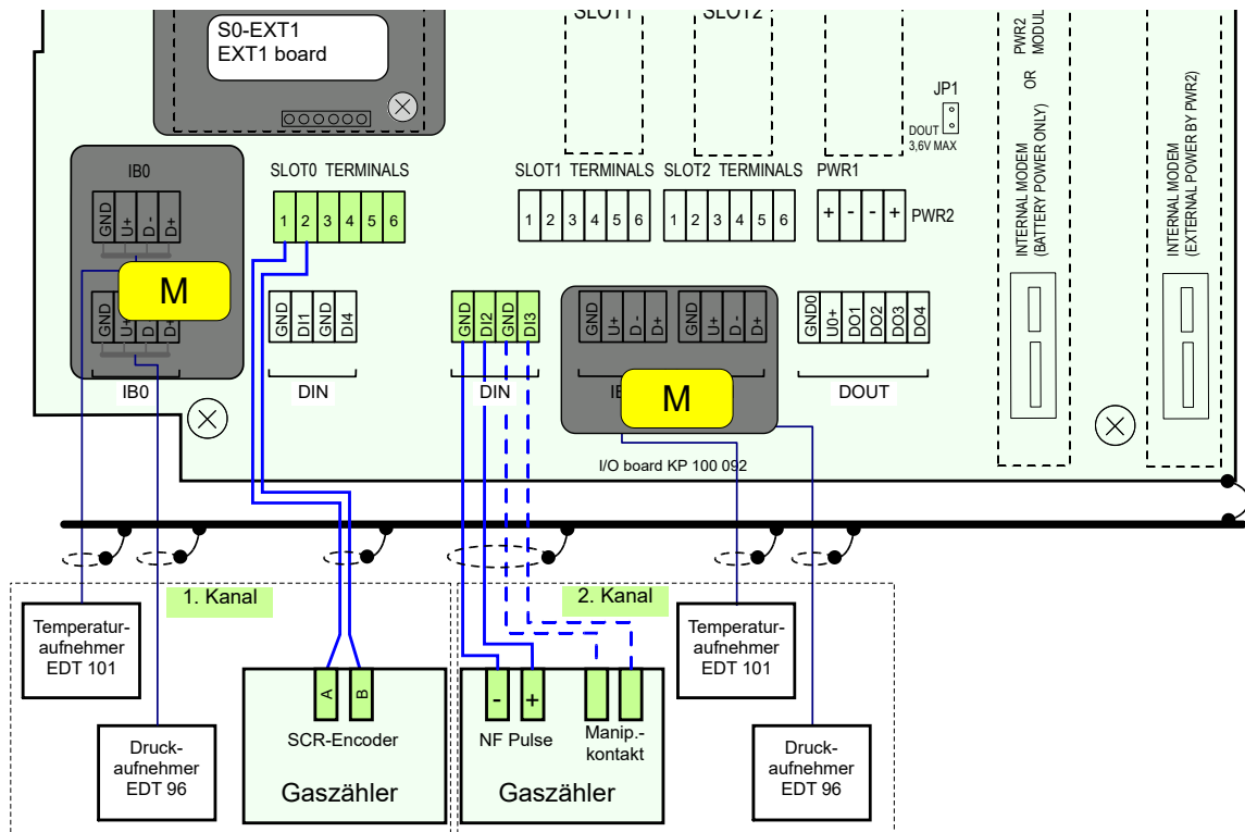
Abb. 15: Anschließen des Gaszählers mit SCR-Encoder am Prilog 400
