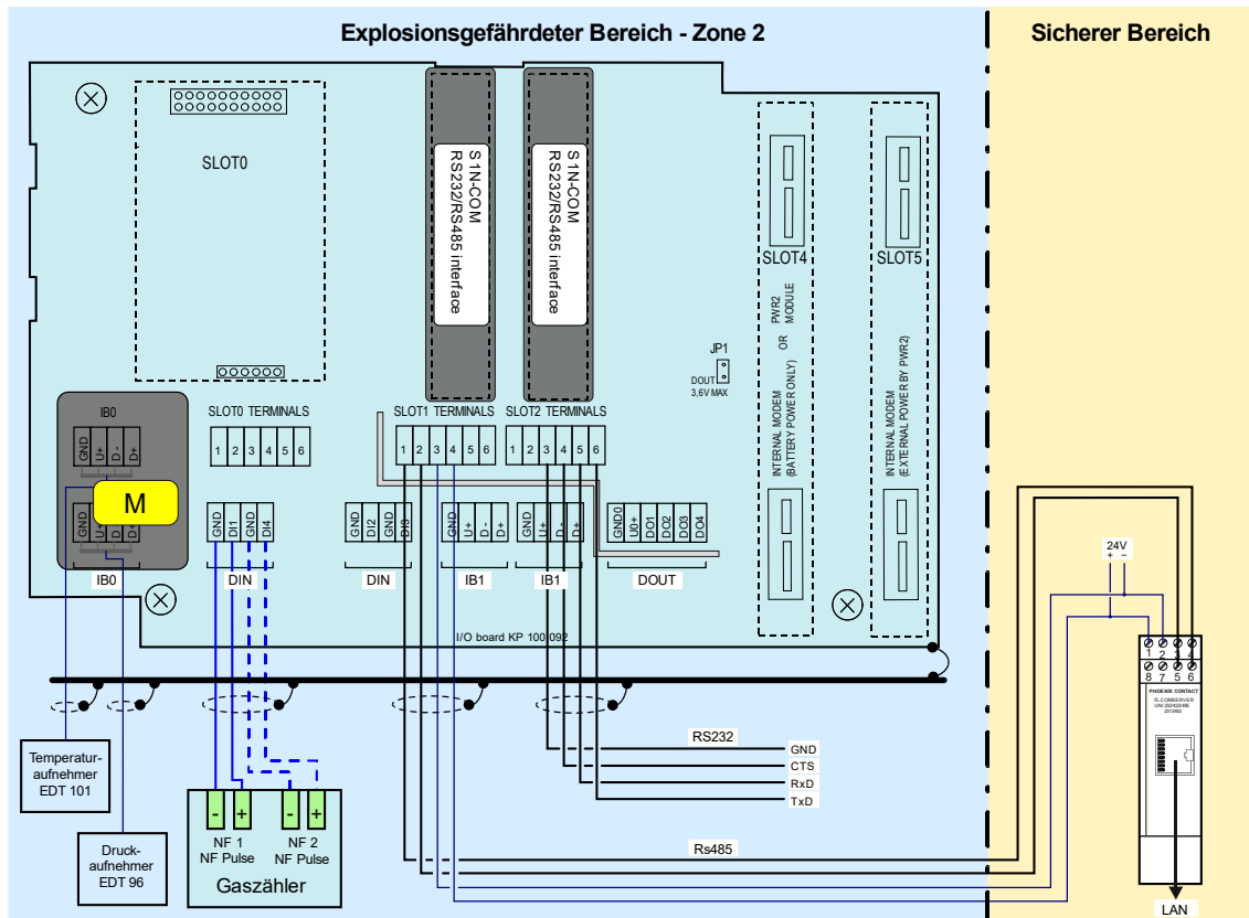
Abb. 59: Prilog 400, Anschluss an LAN über RS485 und Comserver
