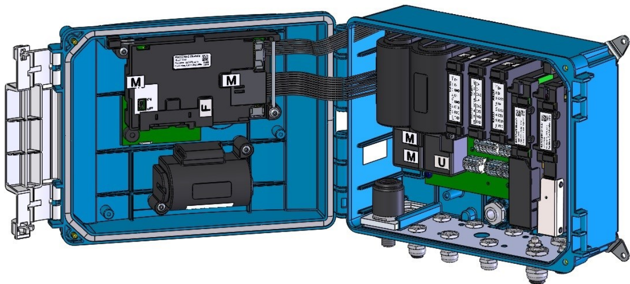
Abb. 2: Innere Sicherheitsmarken des Prilog 400
