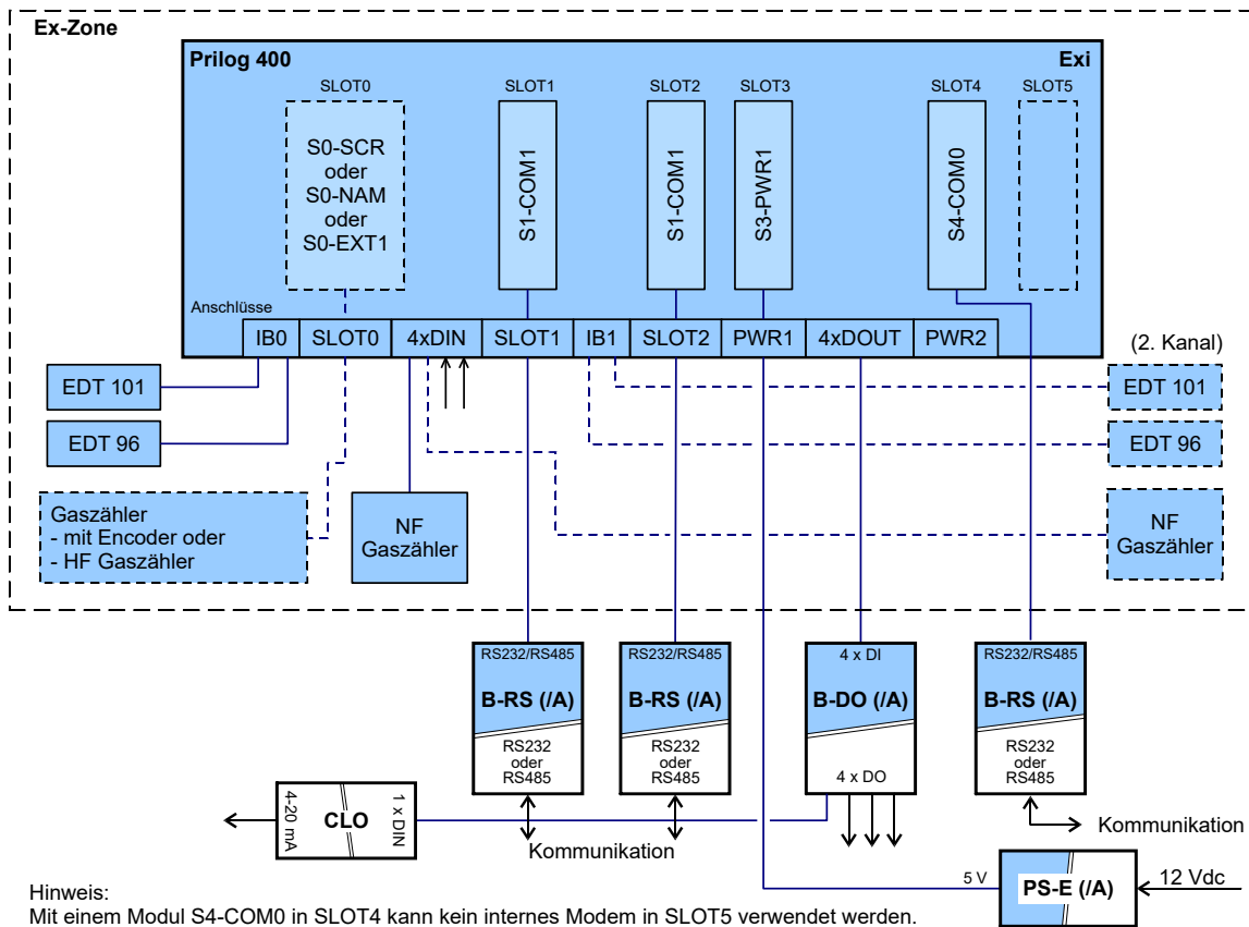
Abb. 54: Prilog 400, Verwendungsbeispiel 2 für externe Module
