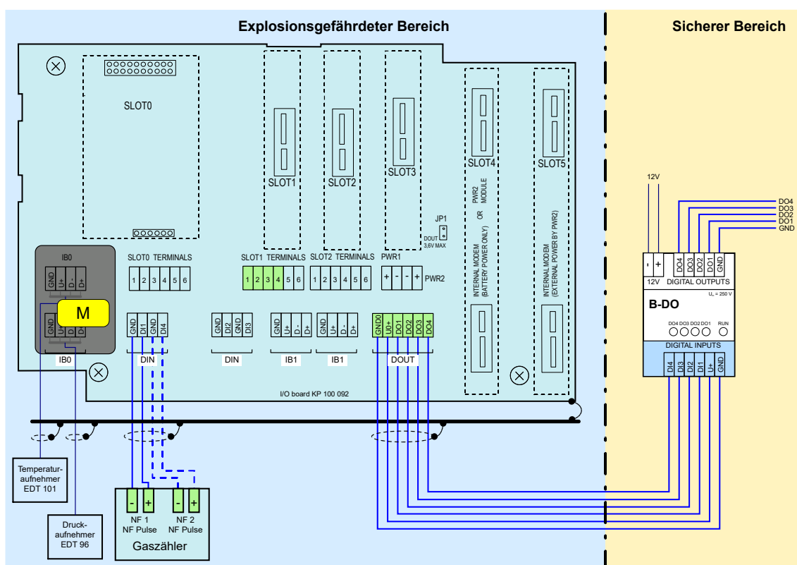
Abb. 16: Anschließen der Digitalausgänge über die Trennbarriere B-DO (Prilog 400)
