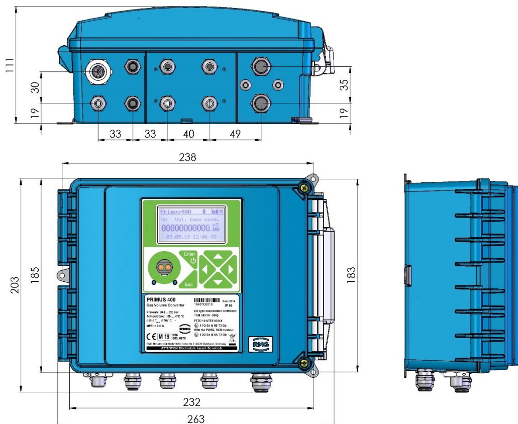
Abb. 1: Prilog 400 Geräteabmessungen
