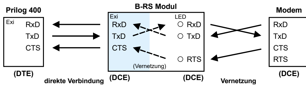
Abb. 45: Anschlussprinzip mit PC und externem Modem über das Modul B-RS
