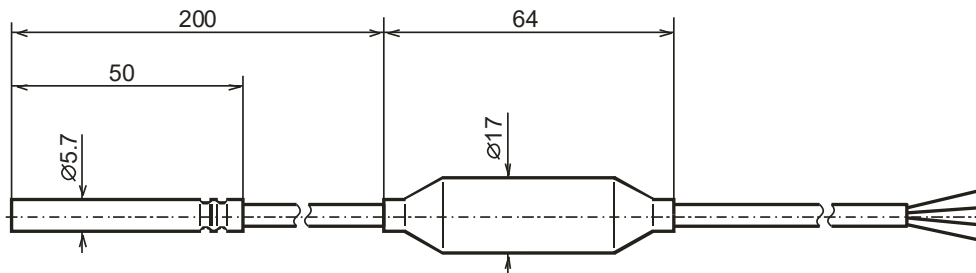
Abb. 42: Sensorabmessungen
