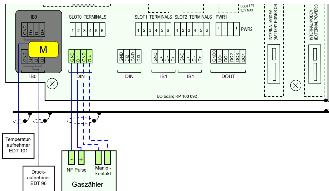
Abb. 12: Anschließen des NF-Gaszählers am Prilog 400 (Einkanal)
