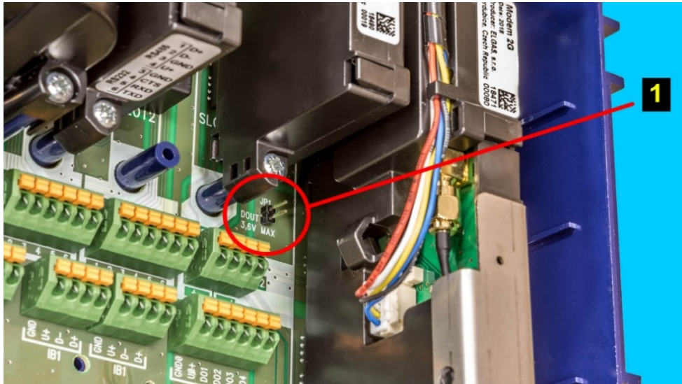
Abb. 40: Installation der Brücke JP1 auf der E/A-Karte
