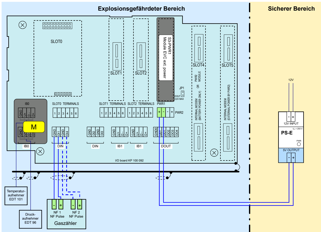
Abb. 19: Anschließen der externen Spannungsversorgung des Messwertregistriergerätes
