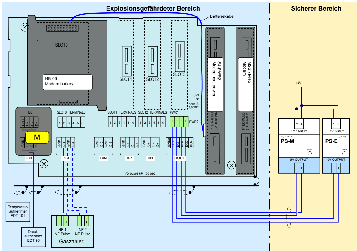
Abb. 21: Externe Spannungsversorgung des Messwertregistriergeräts und des internen Modems
