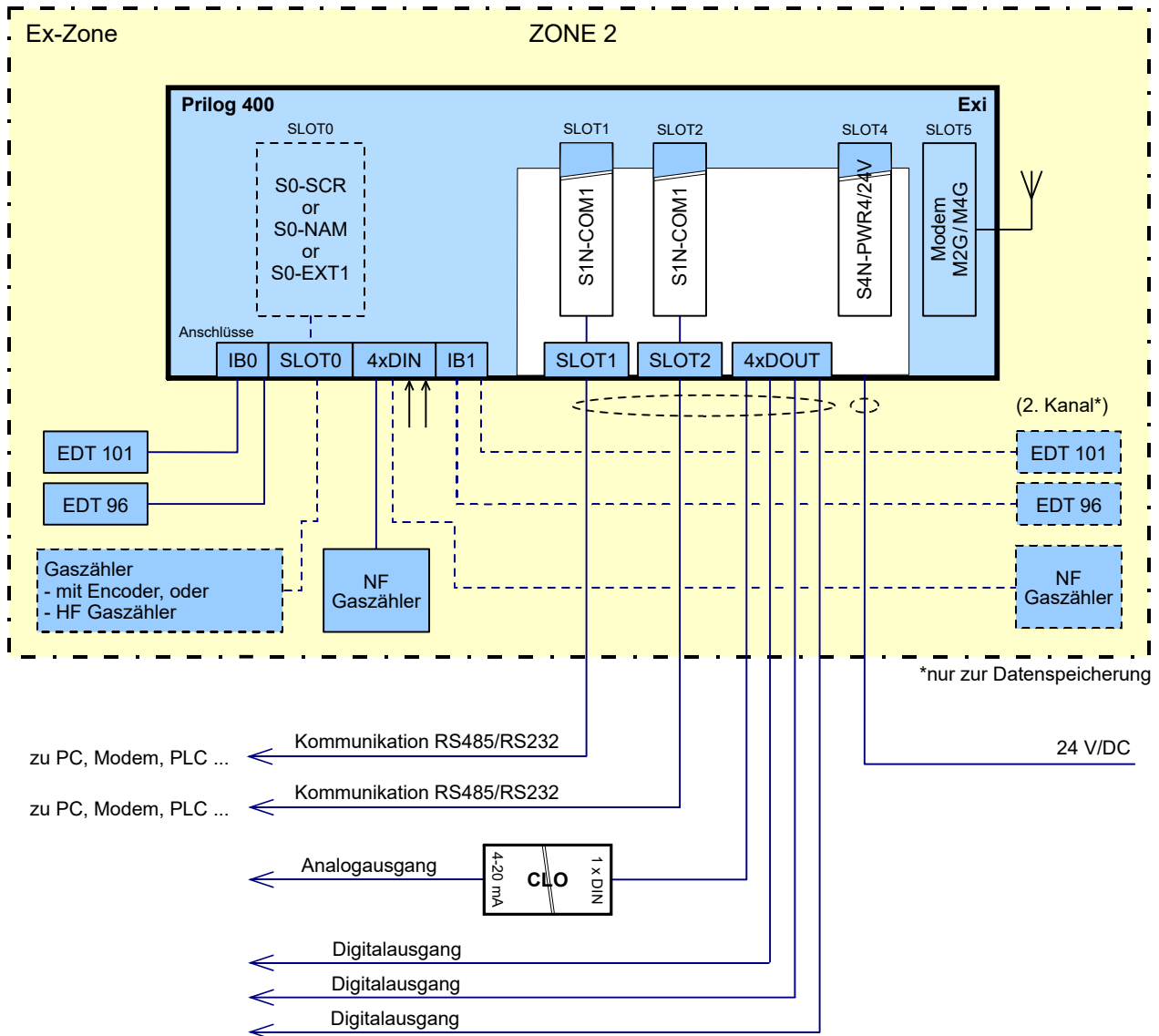
Abb. 60: Blockschaltbild, Prilog 400 für Zone 2 mit ext. 24V Spannungsversorgung
