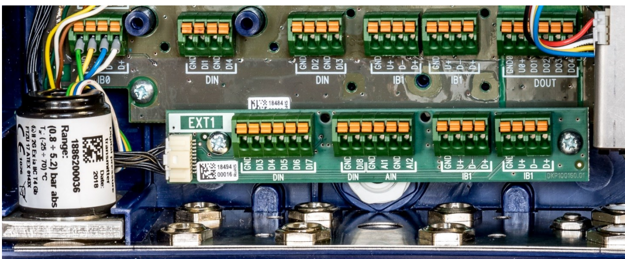
Abb. 44: Zusatzanschlusskarte EXT1-T für das Modul S0-EXT1
