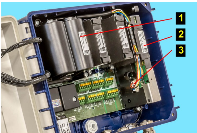
Abb. 25: Anschließen der Modembatterie für Prilog 400
