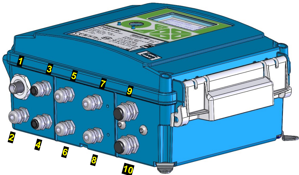
Abb. 56: Anordnung der Kabelverschraubungen
