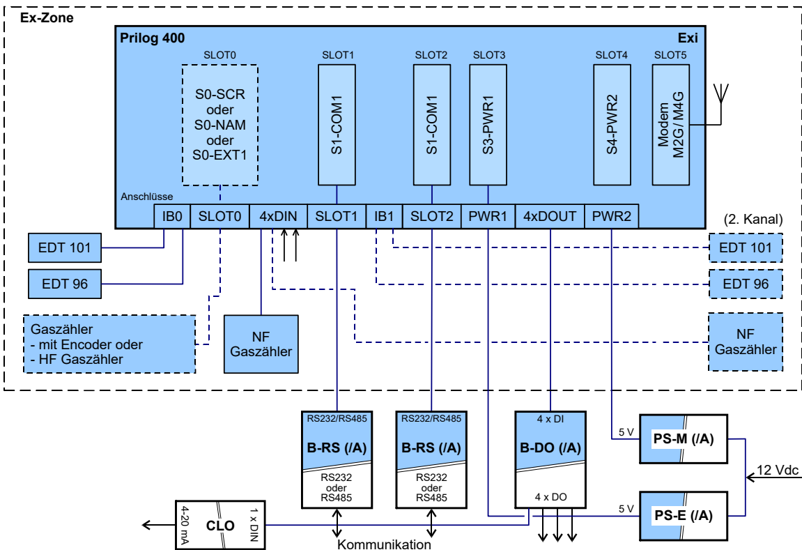
Abb. 53: Prilog 400, Verwendungsbeispiel 1 für externe Module
