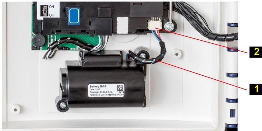
Abb. 24: Anschließen der Gerätebatterie
