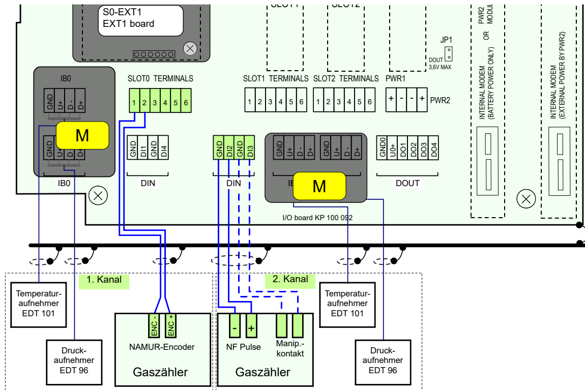
Abb. 14: Anschließen des Gaszählers mit NAMUR-Encoder am Prilog 400
