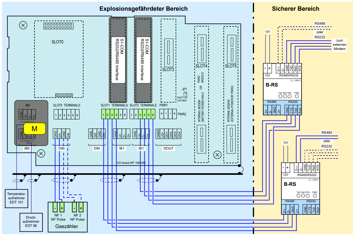
Abb. 22: Prilog 400, Kommunikation über zwei unabhängige Schnittstellen RS232/RS485
