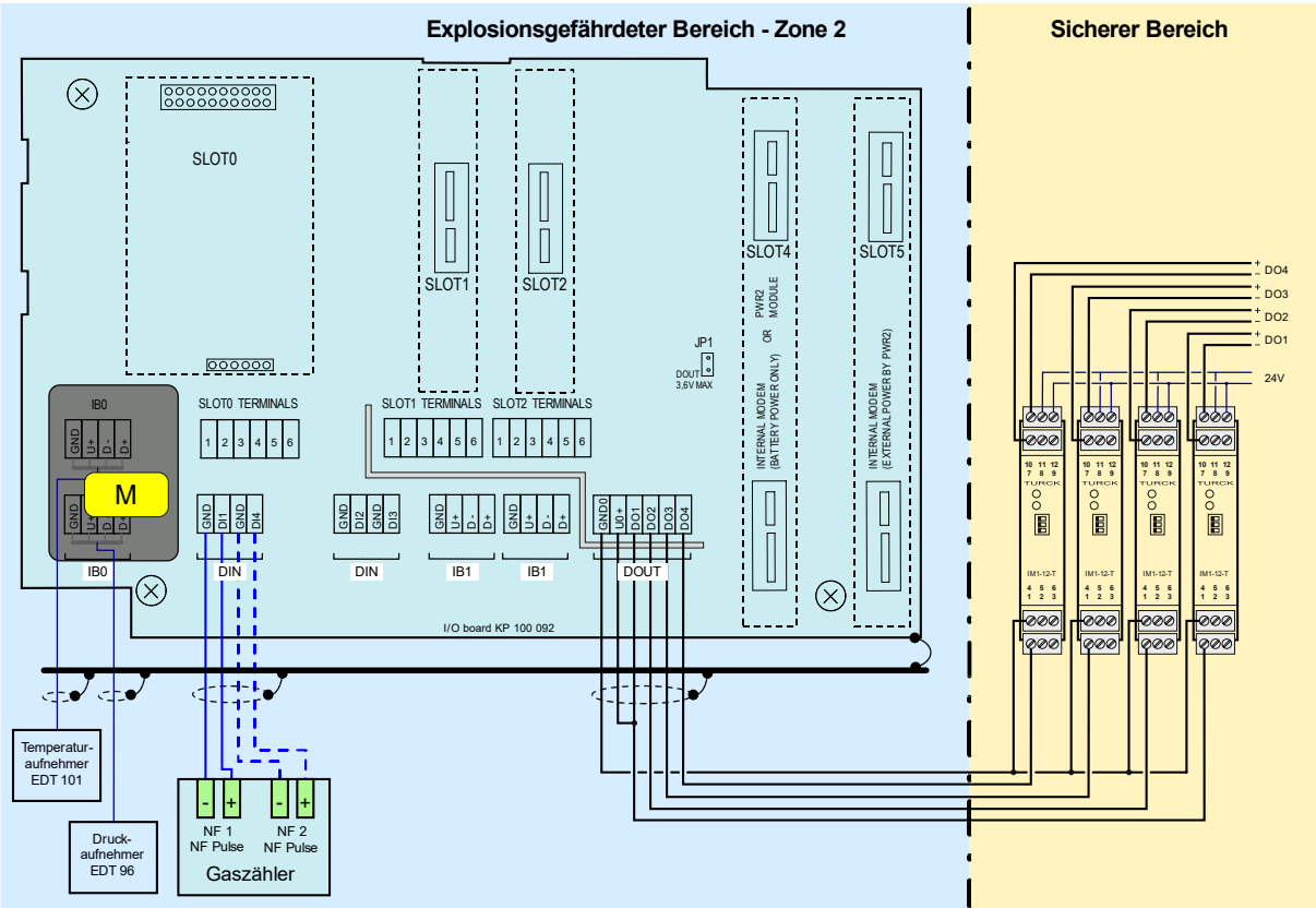
Abb. 58: Anschließen der Digitalausgänge über die Trennbarrieren IM1-12-T (Prilog 400)
