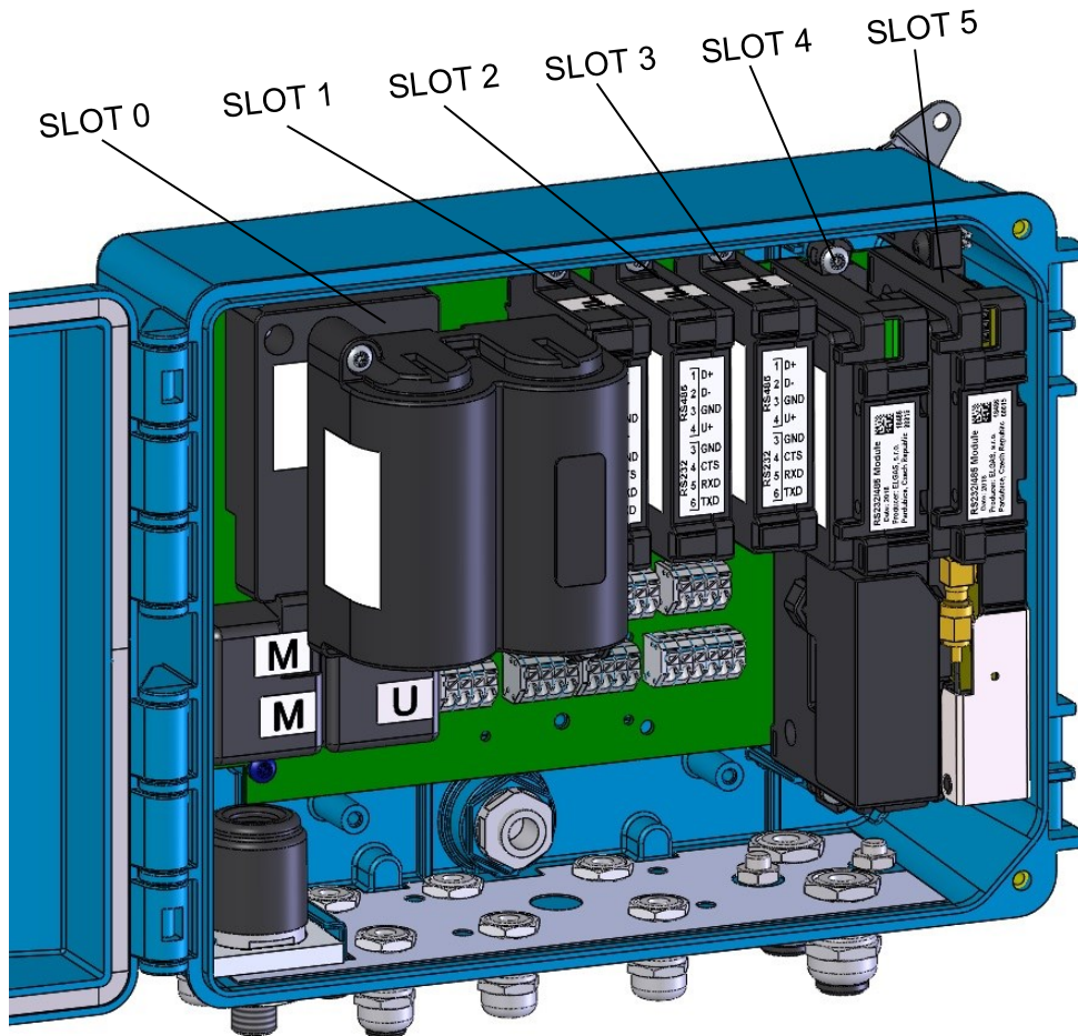
Abb. 37: Anordnung der Steckplätze (Slots) des Prilog 400
