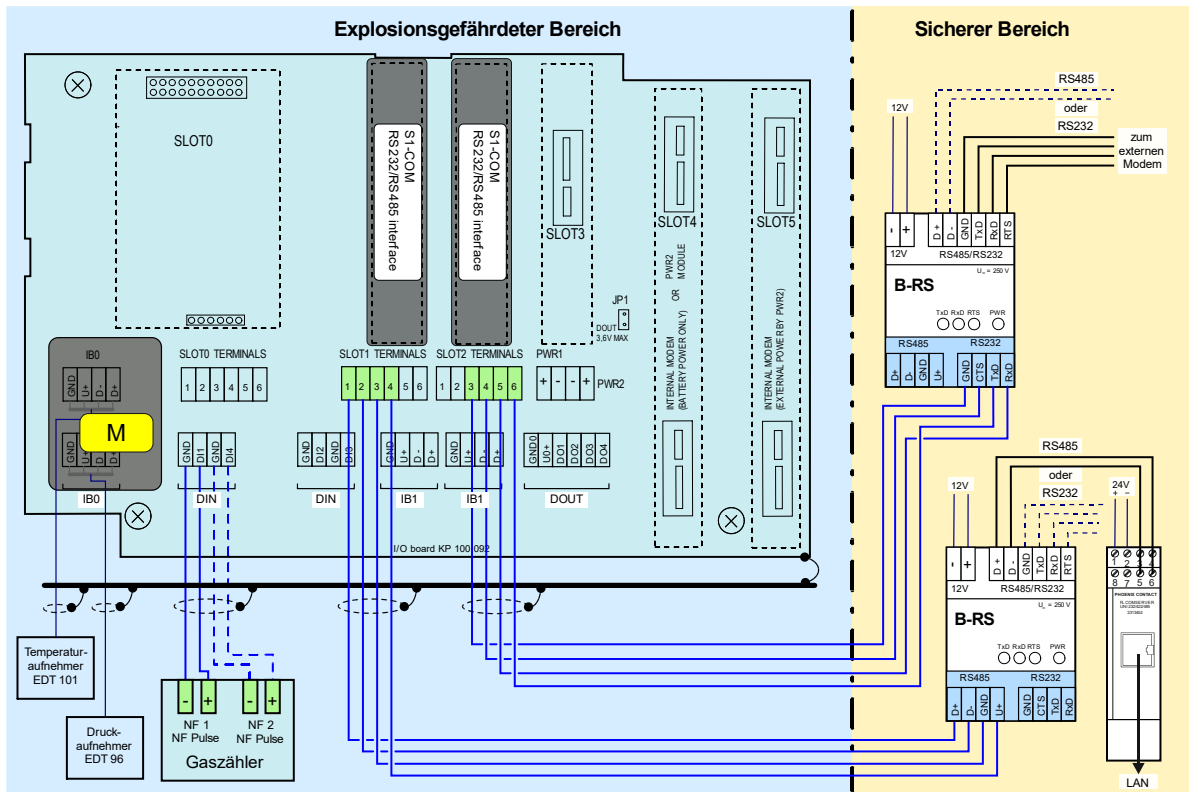
Abb. 23: Prilog 400, Anschluss an RS232 sowie an LAN über RS485 und Comserver
