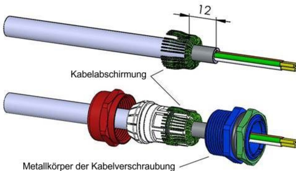
Abb. 10: Verbindung der Kabelabschirmungen in den Kabelverschraubungen
