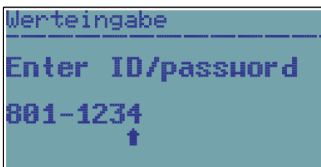
Abb. 52: Passworteingabe
