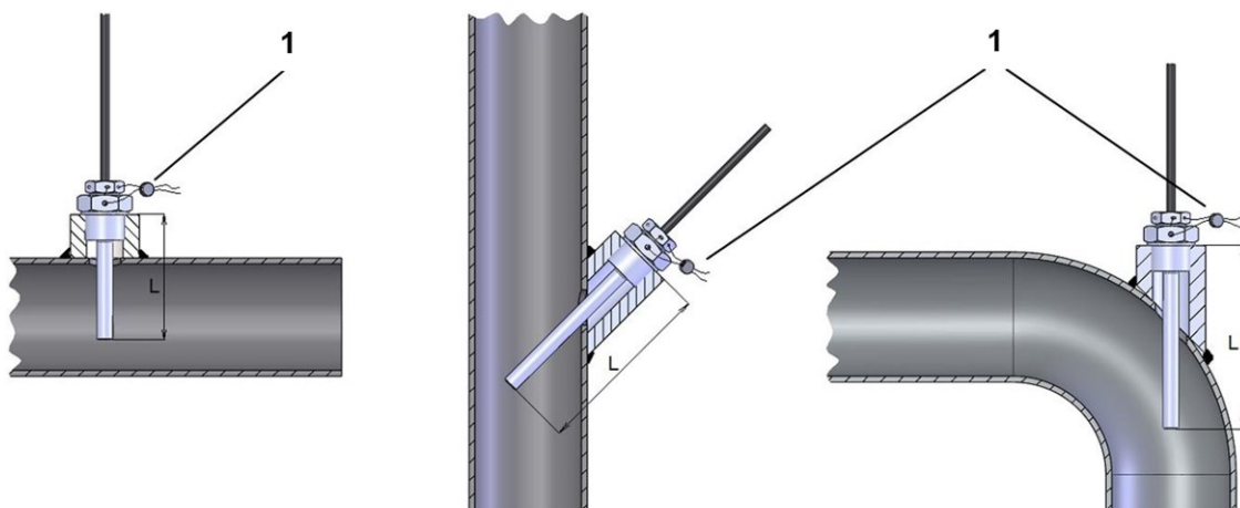
Abb. 8: Montage des Temperatursensors an der Gasleitung
