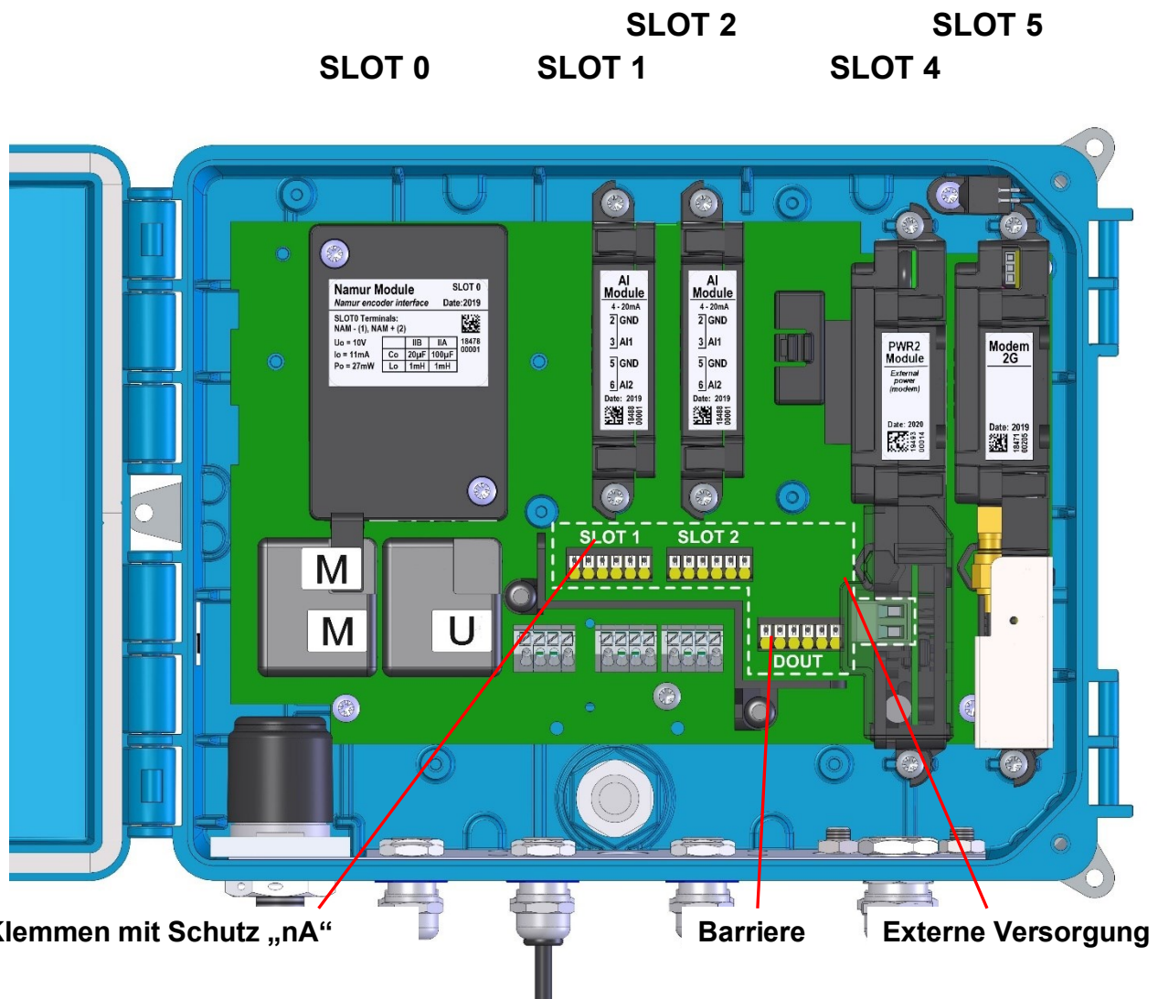
Abb. 55: Klemmen mit Schutz „nA“
