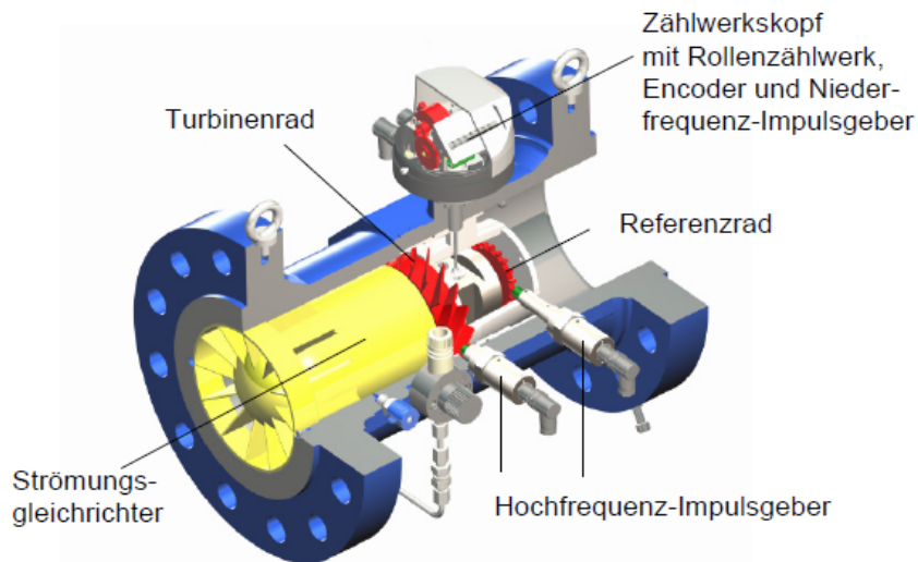
Abbildung 71: Schnittzeichnung RMG Turbinenradgaszähler
