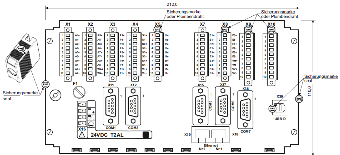
Abbildung 3: Plombenplan Seiten A, B, C, D
