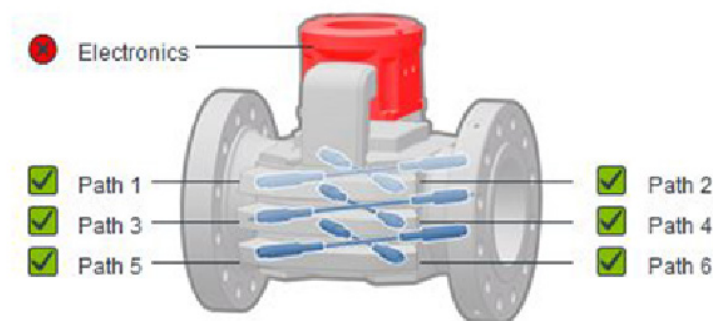
Abbildung 73: Messpfadanordnung USM-GT400
