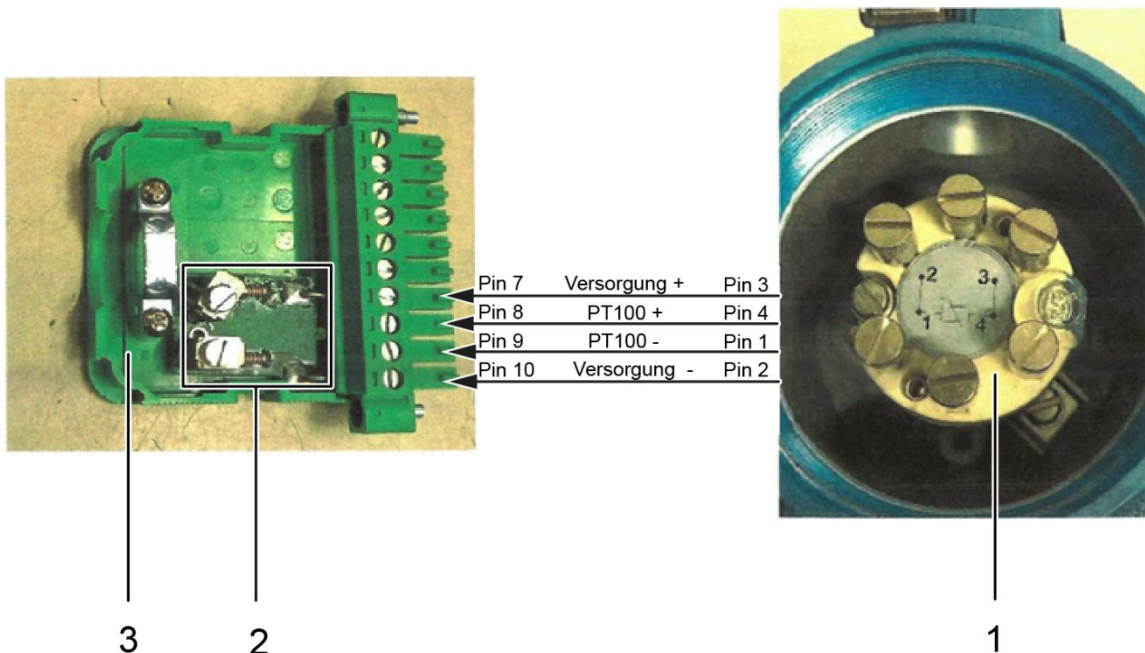
Abbildung 67: Anschluss eines PT100 ohne Vorwiderstände an einen Anschlussstecker
